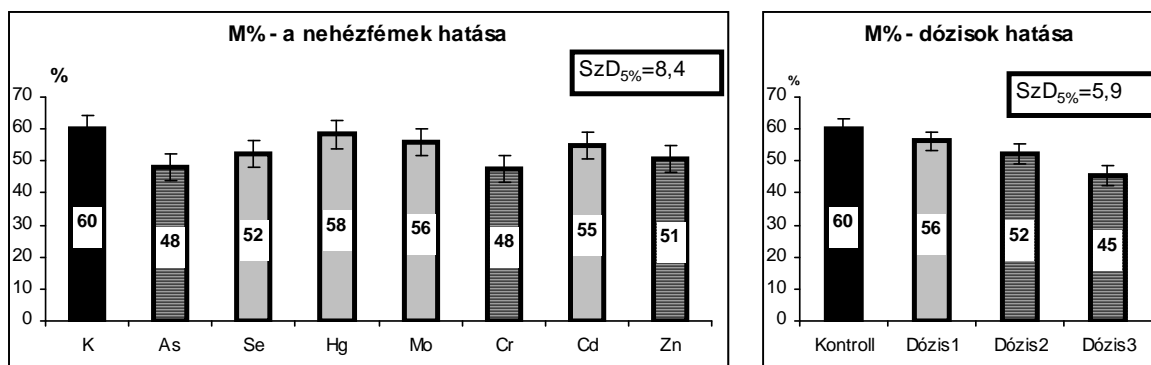
1. ábra: A mikorrhiza gombák infekciójának intenzitása (M%) 14-évi tartamhatású nehézfémek (As, Se, Hg, Mo, Cr, Cd és Zn) és dózisaik (0, 30, 90, 270 mg.kg -1 sz. talaj) hatására lucerna ( Medicago sativa ) gyökérrendszerében szabaföldi kísérletben (Nagyhorcsök, 2005). Megjegyzés: a vízszintes sraffozás szignifikáns különbséget jelöl.
