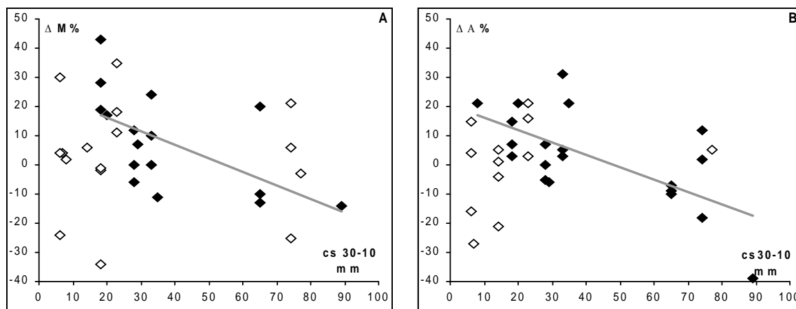
11. ábra: A mikorrhizációs kolonizáció változása ( \square M\% , \square A\% ) és a csapadékmennyiség (cs30-10 – a mintavételt megelőző 30. naptól a mintavételt megelőző 10. napig hullott csapadék) közötti korrelációs összefüggések: A: az M%-ra vonatkozó negatív korreláció az április-július adatsorra áll fenn ( n=24 , R=-0,71 ). B: az arbuszkulumokra (A%) vonatkozó korreláció az április-augusztus adatsorra áll fenn ( n=20 , R=-0,65 ). A korreláció p=0,01 szinten szignifikáns.
