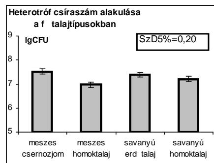
6. ábra: A heterotróf összcsíraszám (telepképz egységek száma, logCFU) alakulása 1 g száraz talajra vonatkoztatva kommunális (Zn-tartalmú) és ipari (Cr-tartalmú) szennyvíziszap-adagok (0, 2,5, 5, 10 és 20 mg.kg -1 ) és különböző talajok (meszes csernozjom és homok, savanyú erd és homok) hatására tenyészedény-kísérletben (Budapest, 2006).
