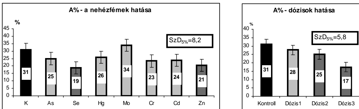
2. ábra: A mikorrhizás arbuszkulum gazdagság (A%) alakulása 14-évi tartamhatású nehézfémek (As, Se, Hg, Mo, Cr, Cd és Zn) és dózisaik (0, 30, 90, 270 mg.kg -1 sz. talaj) hatására lucerna ( Medicago sativa ) gyökérrendszerében, szabaföldi kísérletben (Nagyhorcsök, 2005). Megjegyzés: a vízszintes sraffozás szignifikáns különbséget jelöl.
