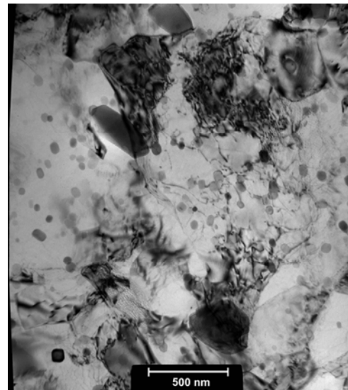
11. ábra Könyöksajtolt ( 1 átnyomás) + 3x50%-os fogyással hengerelt AlMgSi1 anyag hosszirányú mikroszerkezeti képe
