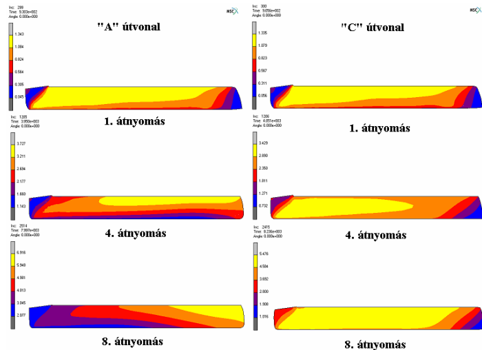
4. ábra Az alakítási út hatása a deformáció eloszlásra (VE modellezés)
