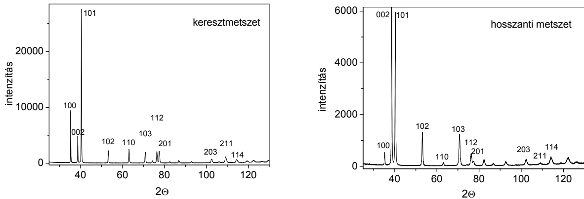
14. ábra A kiindulási minta keresztmetszetéről és hosszanti metszetéről készült röntgen diffraktogramok
