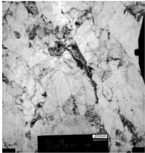
16. ábra Könnyősajtolással +radiális kovácsolással alakított minta a) hosszirányú és b) keresztmetszeti elektronmikroszkópos képe. .
