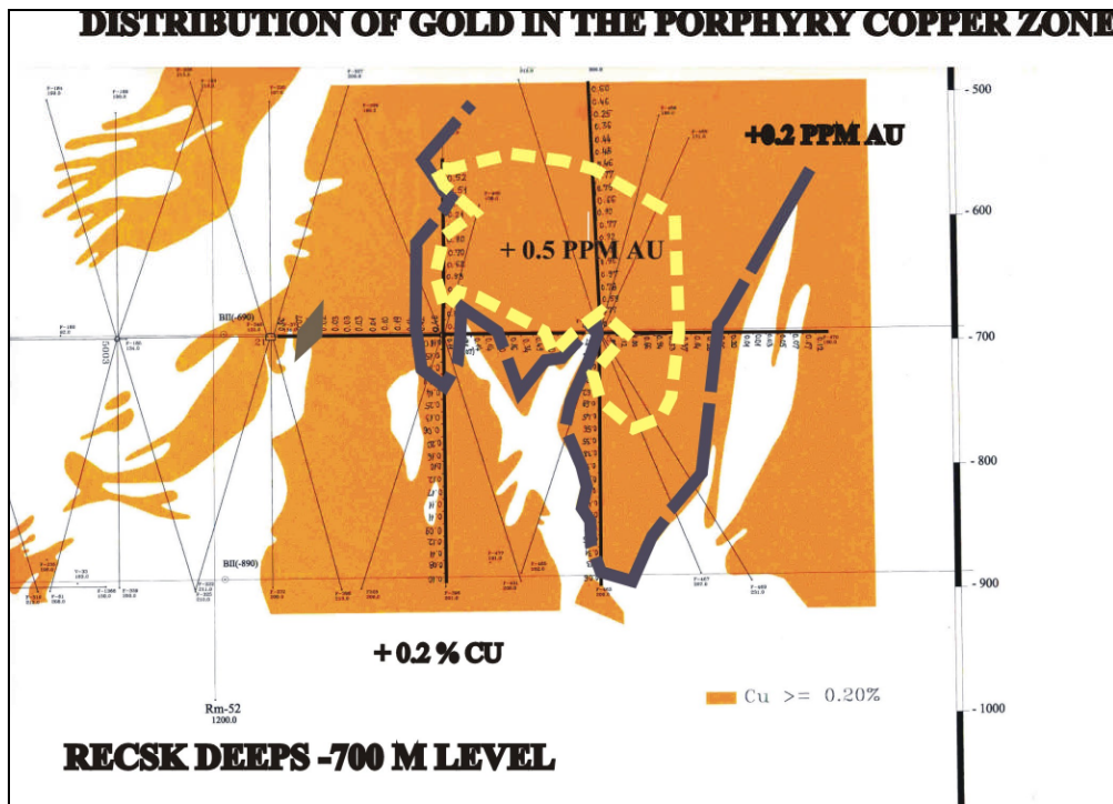
Arany koncentráció eloszlása a recski mélyszínten, két különböző korú diorit kontaktusán
