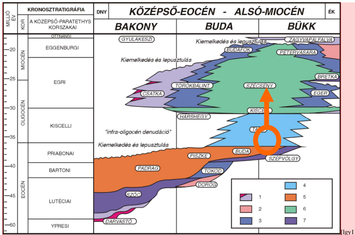
A recski vulkanizmus korának új modellje radiometrikus kor és őslénytani vizsgálatok alapján. A kör a korábbi felfogást, a nyíl a projekt során igazolt kort mutatja
