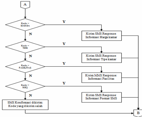
Gambar 3 Flowchart sistem message processing (lanjutan)
