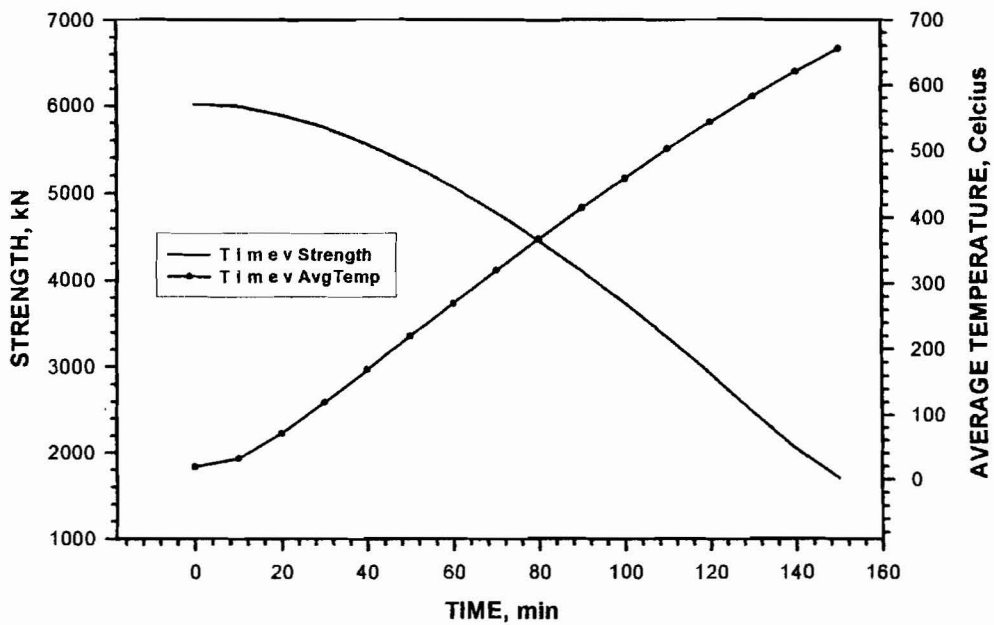
Fig. 14 Column FS3
