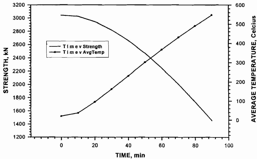
Fig. 12 Column FS1
