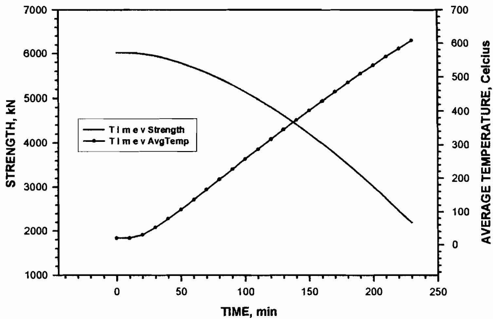
Fig. 16 Column FS5
