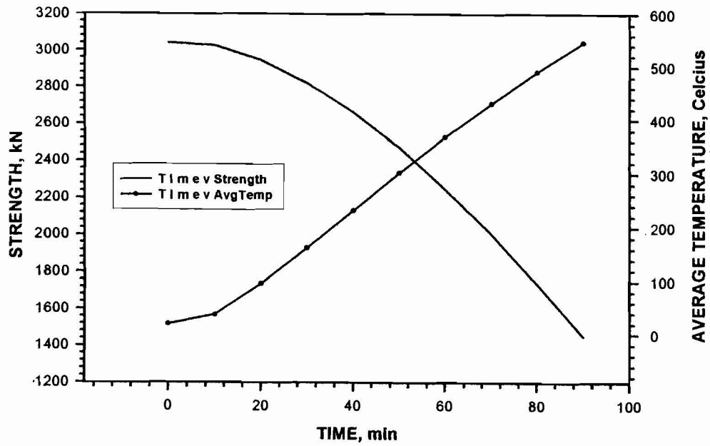
Fig. 15 Column FS4
