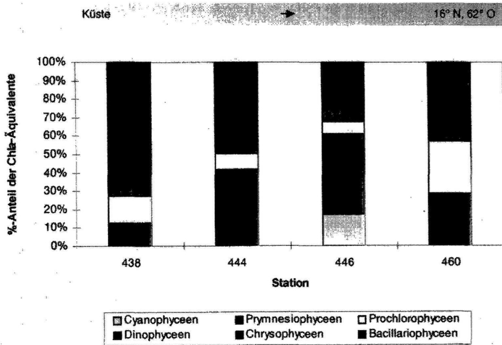
Abb. 4.36 Prozentuale Anteile der Phytoplanktonklassen an den Chl a -Äquivalenten integriert über die oberen 100 m der Wassersäule entlang des Schnittes von der Küste bis 16° N, 62° O während der Expedition METEOR 32/5.
