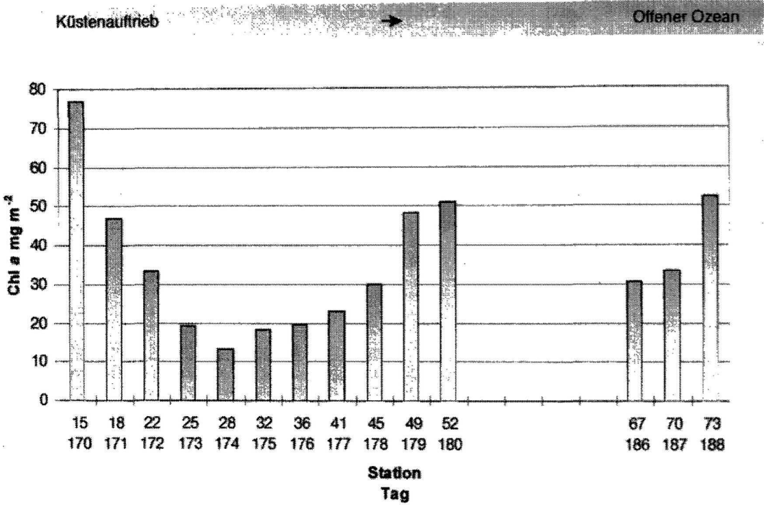
Abb. 5.7 Chl a-Konzentration in mg m -2 integriert über die Tiefe der Sinkstoffalle entlang der Drifttrajektorie während der Expedition SONNE 120.
