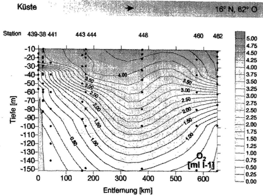
Abb. 4.31 Sauerstoff in \text{ml l}^{-1} in den oberen 150 m der Wassersäule entlang des Schnittes von der Küste bis 16^\circ \text{ N} , 62^\circ \text{ O} während der Expedition METEOR 32/5.
