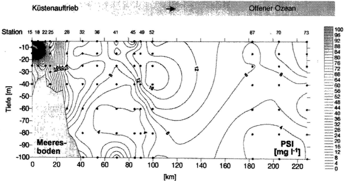
Abb. 5.16 Biogenes partikuläres Silikat (PSi) in \text{mg l}^{-1} in den oberen 100 m der Wassersäule entlang der Drifttrajektorie während der Expedition SONNE 120.
