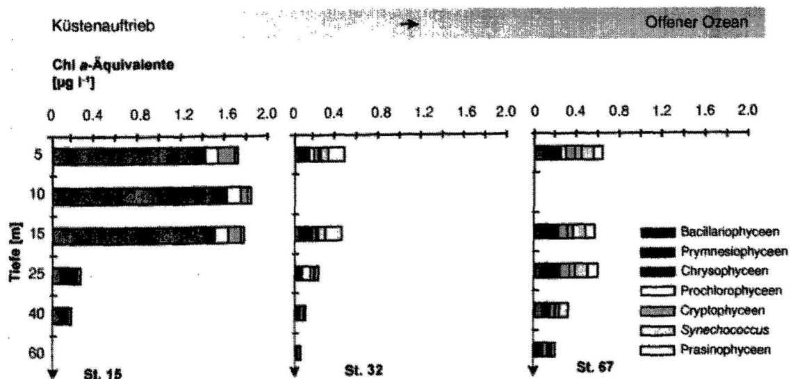
Abb. 5.11 Chl a-Äquivalente der einzelnen Phytoplanktonklassen in \mu\text{g l}^{-1} in den beprobten Tiefen an drei ausgewählten Stationen entlang der Drifttrajektorie während der Expedition SONNE 120.
