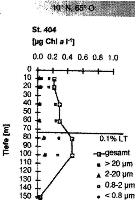
Abb. 4.7 Größenfraktioniertes Chl a in \mu\text{g l}^{-1} in den oberen 150 m der Wassersäule auf St. 404 während der Expedition METEOR 32/5.
