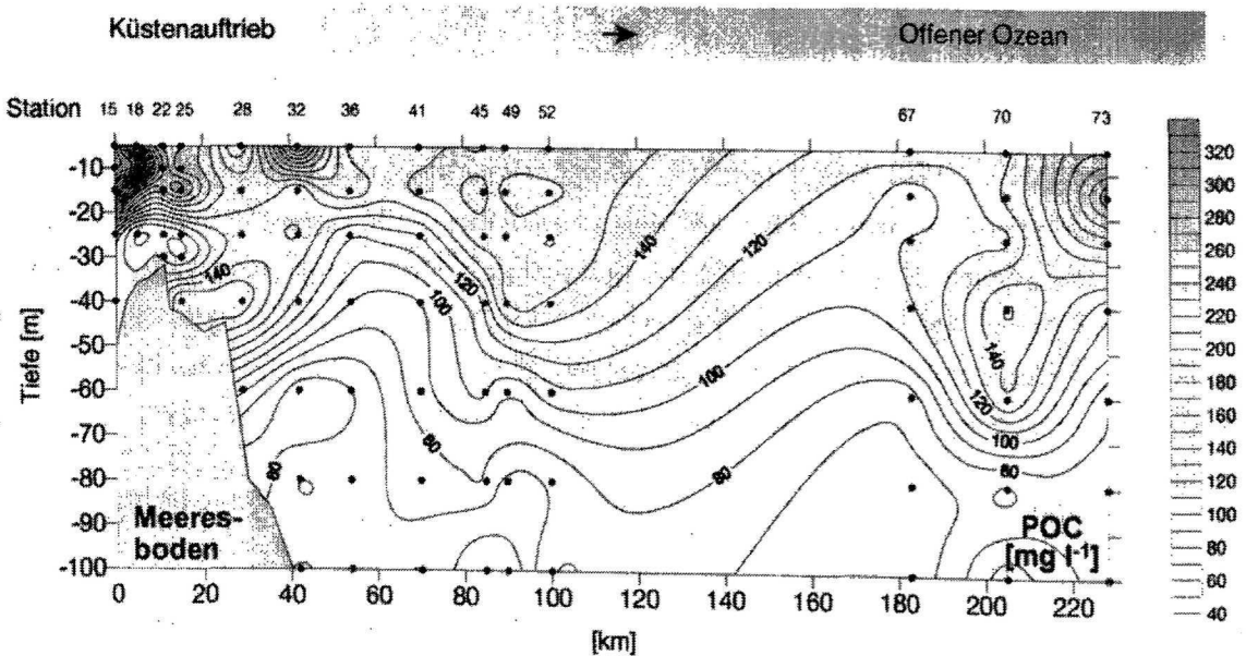
Abb. 5.13 Partikulärer organischer Kohlenstoff (POC) in \text{mg l}^{-1} in den oberen 100 m der Wassersäule entlang der Drifttrajektorie während der Expedition SONNE 120.
