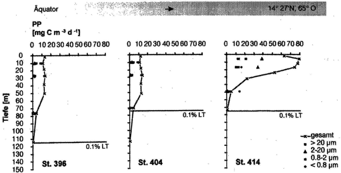
Abb. 4.14 In situ Primärproduktion (PP) der unterschiedenen Größenfraktionen in \text{mg C m}^{-3} \text{d}^{-1} in den verschiedenen Lichttiefen (LT) entlang des Süd-Nord-Schnittes ( 65^\circ \text{O} ) während der Expedition METEOR 32/5.
