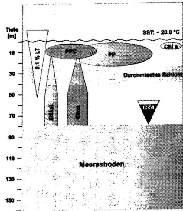
Abb. 8.1 Überblicksdarstellung der drei definierten Regionen des westlichen Arabischen Meeres. SST (Sea Surface Temperature): Oberflächentemperatur; 0.1 % LT (0.1 % Lichttiefe): euphotische Zone; PPC: Phytoplanktonkohlenstoff; PP: Primärproduktion; Chl a: Chlorophyll a; POC: Partikulärer organischer Kohlenstoff, sedimentiert aus der euphotischen Zone. Die Fläche der Symbole bzw. die Breite der Pfeile (Nitrat und Silikat) sind proportional zu ihren Werten.
