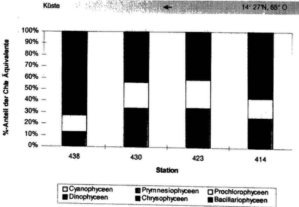
Abb. 4.22 Prozentuale Anteile der Phytoplanktonklassen an den Chl a -Äquivalenten integriert über die oberen 100 m der Wassersäule entlang des Schnittes von 14° 27'N, 65° O bis in den Küstenauftrieb vor Oman während der Expedition METEOR 32/5.
