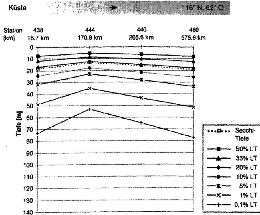
Abb. 4.32 Secchi-Tiefe in m und daraus berechnete Lichttiefen (LT) in m entlang des Schnittes von der Küste bis 16^\circ \text{ N} , 62^\circ \text{ O} während der Expedition METEOR 32/5.
