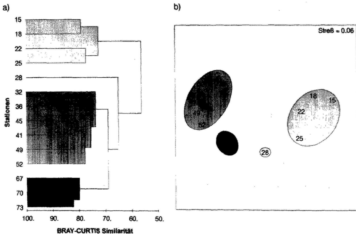
Abb. 5.19 a) Dendrogramm und b) Multidimensionale-Skalierung (MDS) des Phytoplanktondatensatzes während der Expedition SONNE 120. Im MDS-Plot markieren die Kreise die Stationsgruppen aus der Clusteranalyse. Streßfaktor (Streß) = 0.06.
