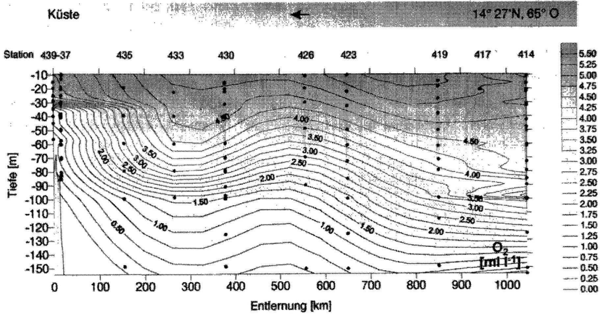
Abb. 4.16 Sauerstoff in \text{ml l}^{-1} in den oberen 150 m der Wassersäule entlang des Schnittes von 14^\circ 27'N, 65^\circ O bis in den Küstenauftrieb vor Oman während der Expedition METEOR 32/5.
