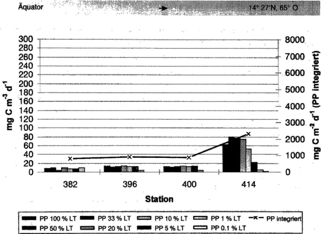
Abb. 4.13 In situ Primärproduktion (PP) des Phytoplanktons in den verschiedenen Lichttiefen (LT) in \text{mg C m}^{-3} \text{d}^{-1} und integriert über die euphotische Zone in \text{mg C m}^{-2} \text{d}^{-1} entlang des Süd-Nord-Schnittes ( 65^\circ \text{O} ) während der Expedition METEOR 32/5.
