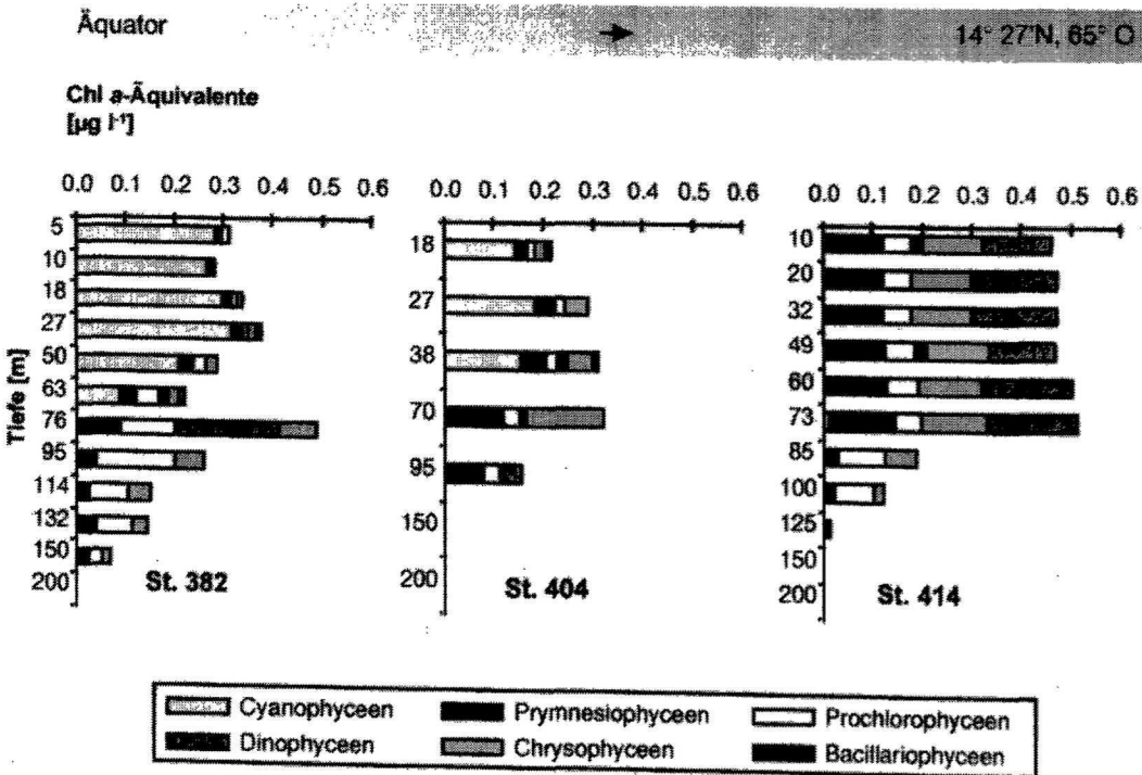
Abb. 4.9 Chl a-Äquivalente in µg l -1 der einzelnen Phytoplanktonklassen in den beprobten Tiefen der St. 382, St. 404 und St. 414 entlang des Süd-Nord-Schnittes (65° O) während der Expedition METEOR 32/5.
