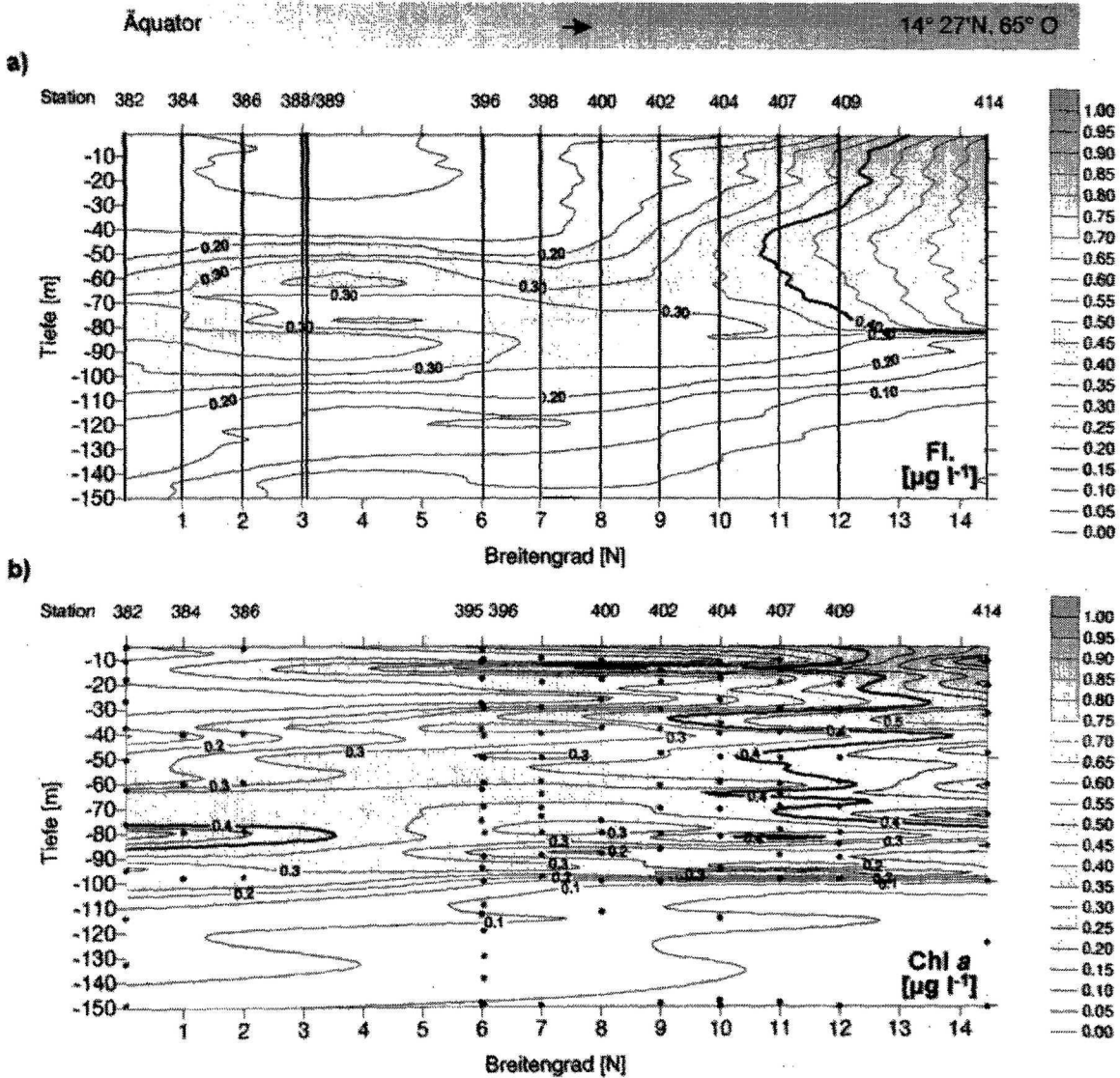
Abb. 4.5a+b in situ Chl a-Fluoreszenz (a) und fluorimetrisch ermittelte Chl a-Konzentration (b) jeweils in \mu\text{g l}^{-1} in den oberen 150 m der Wassersäule entlang des Süd-Nord-Schnittes (65° O) während der Expedition METEOR 32/5.
