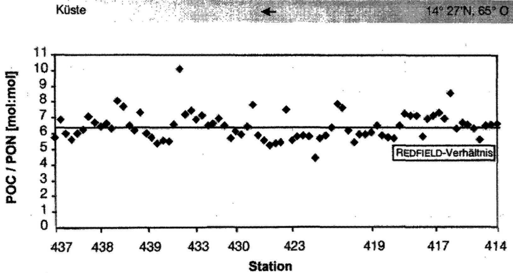
Abb. 4.25 Das molare C:N-Verhältnis entlang des Schnittes von 14^{\circ} 27' \text{ N} , 65^{\circ} \text{ O} bis in den Küstenauftrieb vor Oman während der Expedition METEOR 32/5. Aufgetragen sind für jede Station jeweils alle Meßwerte der oberen 150 m der Wassersäule.
