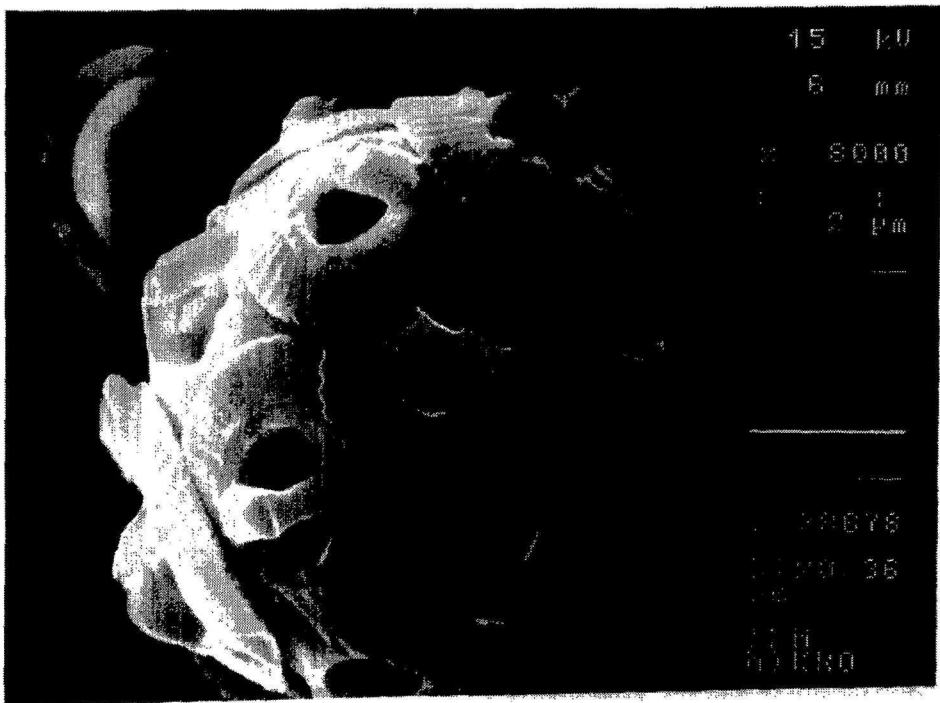
Tafel I Rasterelektronenmikroskopische Aufnahmen der Coccolithophoridenart Gephyrocapsa oceanica .
