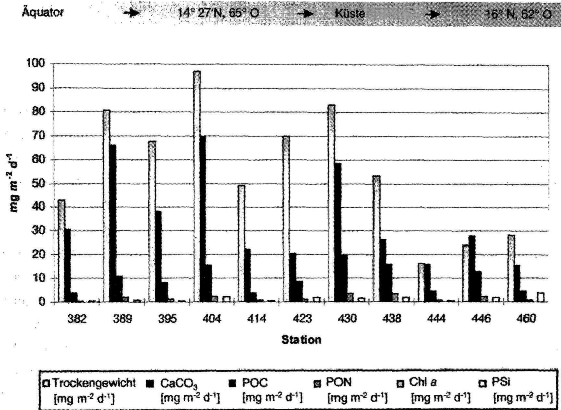
Abb. 4.43 Zusammensetzung des Sinkstoffallenmaterials (Trockengewicht, TG, und dessen Hauptkomponenten) in \text{mg m}^{-2} \text{d}^{-1} für den gesamten Untersuchungszeitraum während der Expedition METEOR 32/5. CaCO 3 : Kalziumkarbonat, POC: partikulärer organischer Kohlenstoff, PON: partikulärer organischer Stickstoff, Chl a: Chlorophyll a, PSi: partikuläres Silikat.
