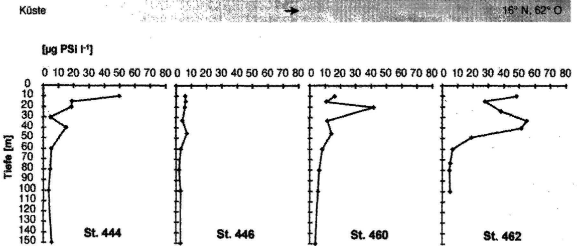
Abb. 4.40 Partikuläres Silikat (PSi) in \mu\text{g l}^{-1} auf St. 444, St. 446, St. 460 und St. 462 entlang des Schnittes von der Küste bis 16^\circ \text{ N} , 62^\circ \text{ O} während der Expedition METEOR 32/5.
