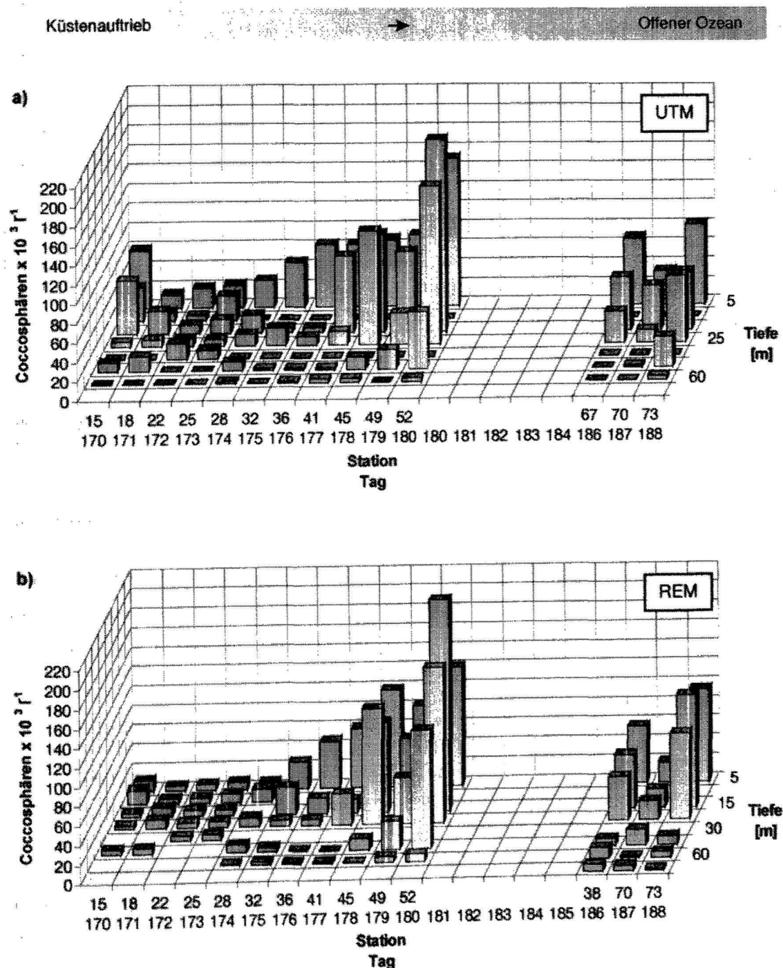
Abb. 5.17a+b Coccolithophoridenzellzahlen [Coccosphären x 10 3 l -1 ] analysiert mittels a) UTERMÖHL- und b) Rasterelektronenmikroskopie (UTM bzw. REM) in verschiedenen Tiefen der euphotischen Zone entlang der Driftrajektorie während der Expedition SONNE 120.
