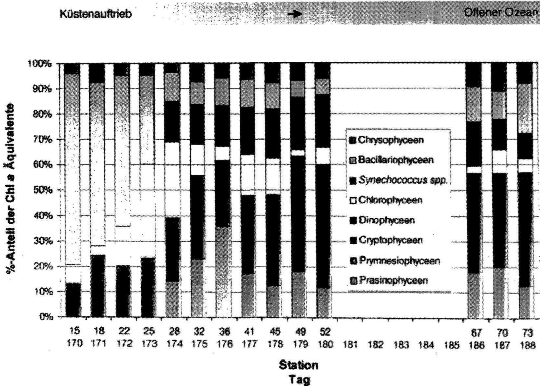
Abb. 5.10 Prozentuale Anteile der Phytoplanktonklassen an den Chl a -Äquivalenten integriert über die jeweilige Tiefe der Sinkstofffalle entlang der Drifttrajektorie während der Expedition SONNE 120.
