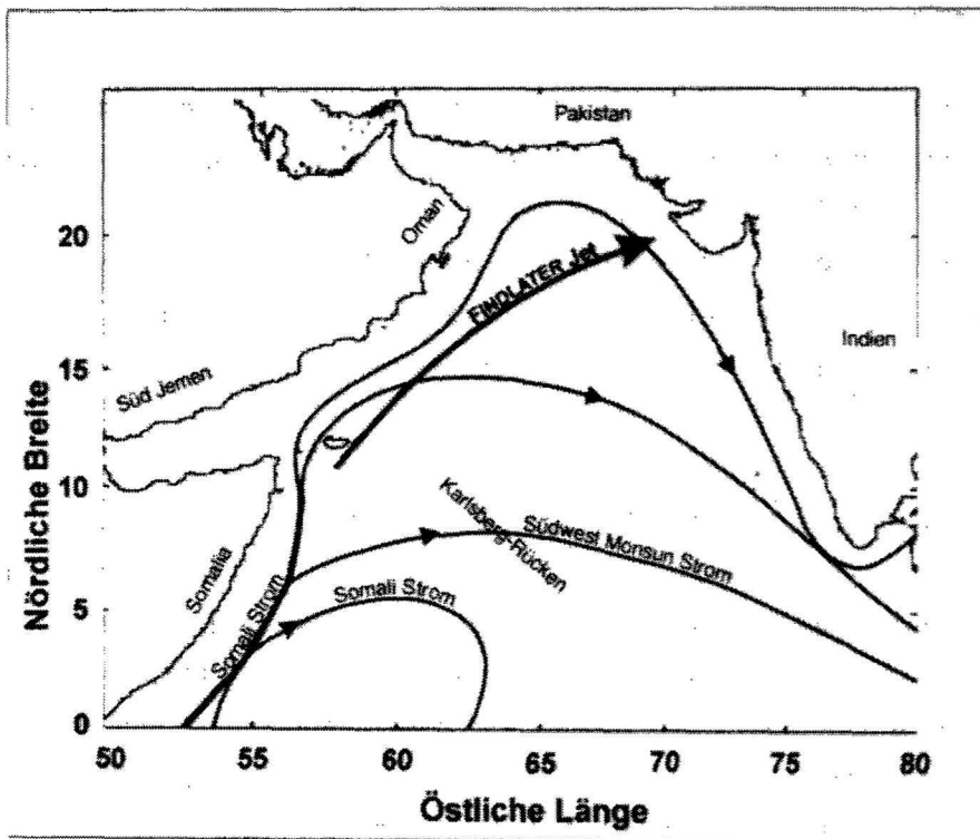
Abb. 2.1 Untersuchungsgebiet während des SW-Monsuns mit schematischem Oberflächenstromsystem (modifiziert nach You, 1997) und dem atmosphärischen Findlater Jet.
