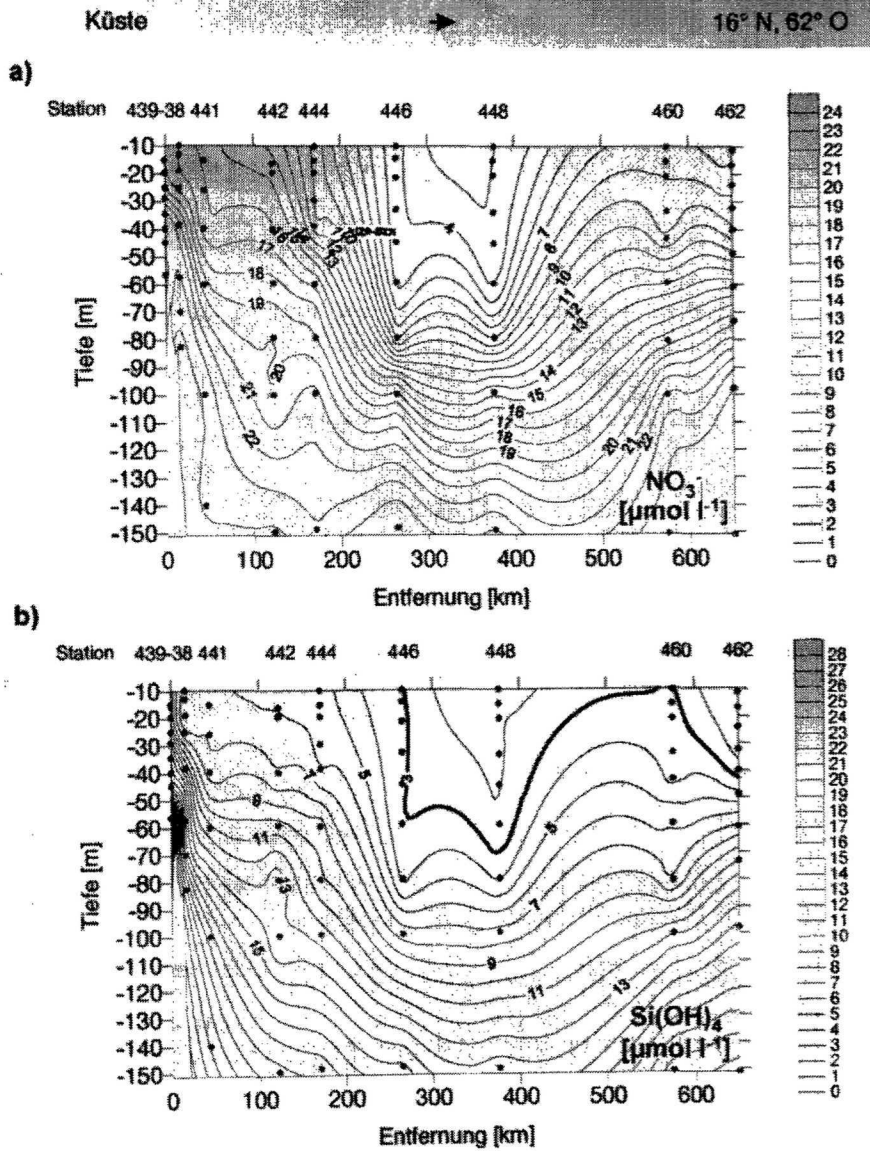
Abb. 4.30a+b Konzentrationen von a) Nitrat und b) Silikat in \mu\text{mol l}^{-1} in den oberen 150 m der Wassersäule entlang des Schnittes von der Küste bis 16^\circ \text{N} , 62^\circ \text{O} während der Expedition METEOR 32/5. b) Die 3 \mu\text{mol l}^{-1} Silikat-Isoplethe ist fettgedruckt.
