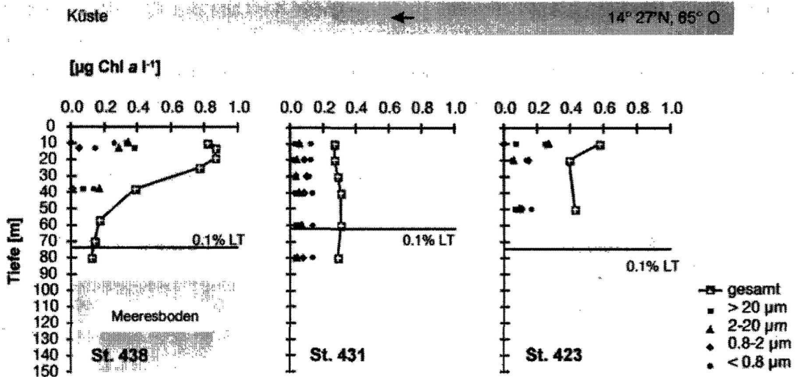
Abb. 4.21 Größenfraktioniertes Chl a in \mu\text{g l}^{-1} in den oberen 150 m der Wassersäule auf St. 423, St. 431 und St. 438 entlang des Schnittes von 14^{\circ} 27' \text{N} , 65^{\circ} \text{O} bis in den Küstenauftrieb vor Oman während der Expedition METEOR 32/5.
