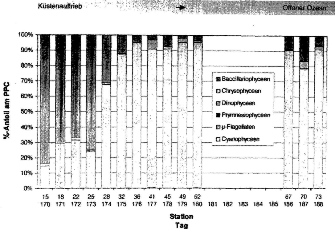
Abb. 5.12 Prozentuale Anteile der Phytoplanktongruppen (UTERMÖHL-Mikroskopie) am Phytoplanktonkohlenstoff (PPC) integriert über die jeweilige Tiefe der Sinkstoffalle entlang der Drifttrajektorie während der Expedition SONNE 120.
