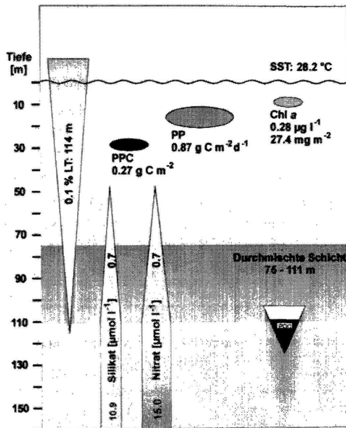
Abb. 7.2 Das Epipelagial des zentralen Arabischen Meeres hinsichtlich seiner physikalischen, chemischen und biologischen Merkmale (Mittelwerte) zur Zeit des SW-Monsuns. SST (Sea Surface Temperature): Oberflächentemperatur; 0.1 % LT: 0.1 % Lichttiefe, euphotische Zone; PPC: Phytoplanktonkohlenstoff; PP: Primärproduktion; Chl a: Chl a in der durchmischten Schicht [ \mu\text{g l}^{-1} ] und integriert über die Tiefe der Sinkstoffalle (100 m) [ \text{mg m}^{-2} ]; POC: Partikulärer organischer Kohlenstoff, sedimentiert aus der euphotischen Zone.
