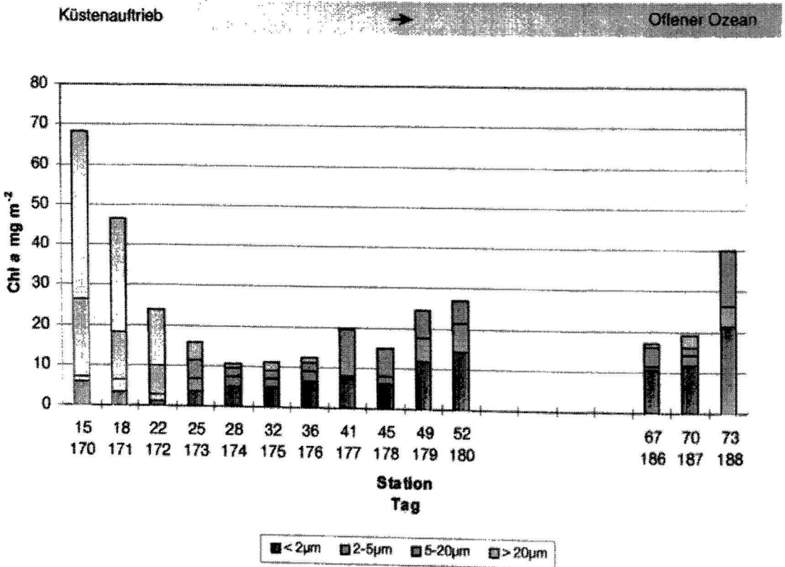
Abb. 5.8 Größenfraktionierte Chl a-Konzentration in mg m -2 integriert über die oberen 25 m der Wassersäule entlang der Drifttrajektorie während der Expedition SONNE 120.
