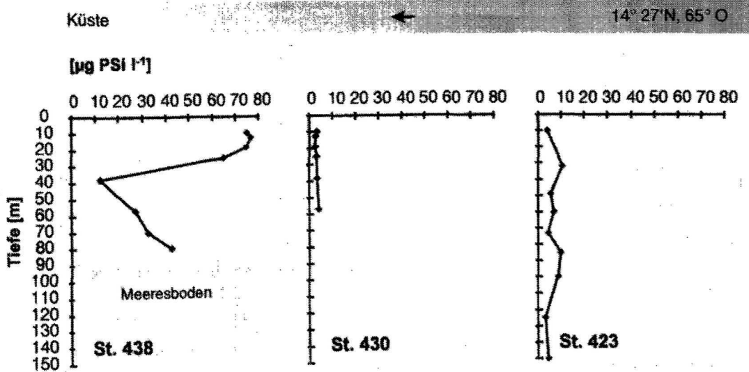
Abb. 4.26 Partikuläres Silikat (PSi) in \mu\text{g l}^{-1} auf St. 423, St. 430 und St. 438 entlang des Schnittes von 14^{\circ} 27' \text{ N} , 65^{\circ} \text{ O} bis in den Küstenauftrieb vor Oman während der Expedition METEOR 32/5.
