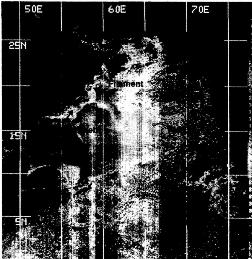
Abb. 2.2 Satellitenaufnahme der Oberflächentemperatur (engl. SST, Sea Surface Temperature, in °C, Legende rechts) des Arabischen Meeres vom 4. August 1995. RSMAS: 'Rosenstiel Institute of Marine Science', Miami, Florida. Dunkelgrau: Wolken.
