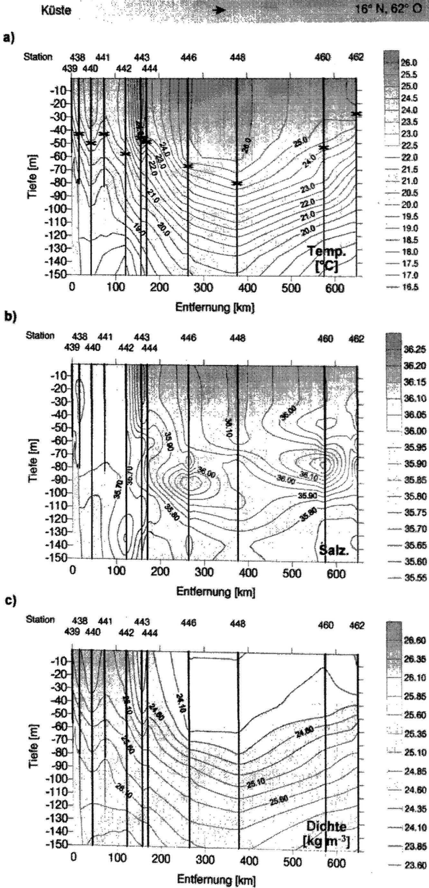
Abb. 4.29a-c Temperatur (a) in °C, Salzgehalt (b) und Dichte (c) in kg m -3 in den oberen 150 m der Wassersäule entlang des Schnittes von der Küste bis 16° N, 62° O während der Expedition METEOR 32/5. a) Die Kreuze markieren die Tiefe der durchmischten Schicht.
