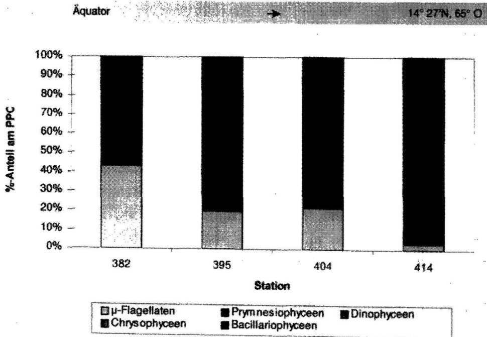
Abb. 4.10 Prozentuale Anteile der Phytoplanktonklassen (UTERMÖHL-Mikroskopie) am Phytoplanktonkohlenstoff (PPC) integriert über die oberen 100 m der Wassersäule entlang des Süd-Nord-Schnittes ( 65^\circ O) während der Expedition METEOR 32/5.
