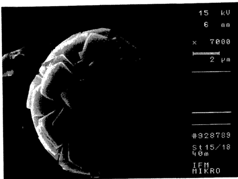
Tafel IIIa Rasterelektronenmikroskopische Aufnahme der Coccolithophoridenart Calciopappus rigidus .
