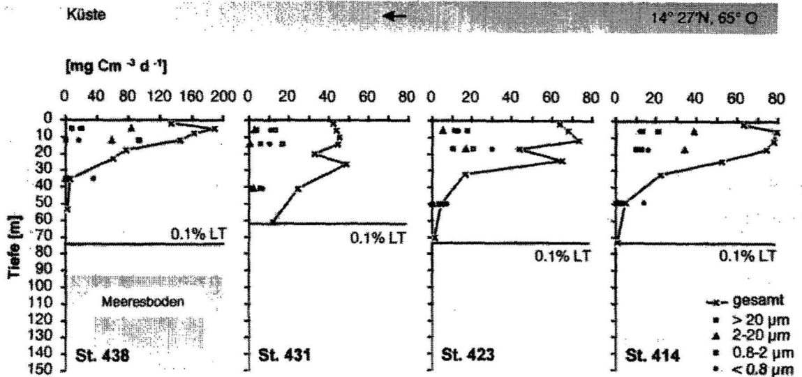
Abb. 4.28 In situ Primärproduktion (PP) der unterschiedenen Größenfraktionen in \text{mg m}^{-3} \text{d}^{-1} in den verschiedenen Lichttiefen (LT) entlang des Schnittes von 14^\circ 27'N, 65^\circ O bis in den Küstenauftrieb vor Oman während der Expedition METEOR 32/5. Aufgrund der hohen Werte im Küstenauftrieb (St. 438) wurde hier eine größere Skala gewählt.
