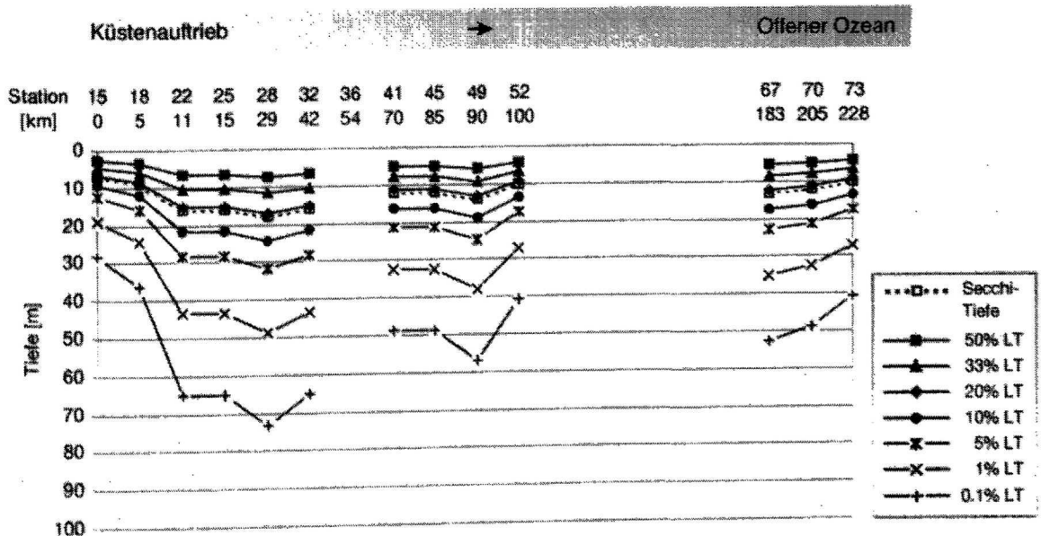
Abb. 5.5 Secchi-Tiefe in m und daraus berechnete Lichttiefen (LT) in m entlang der Drifttrajektorie während der Expedition SONNE 120.
