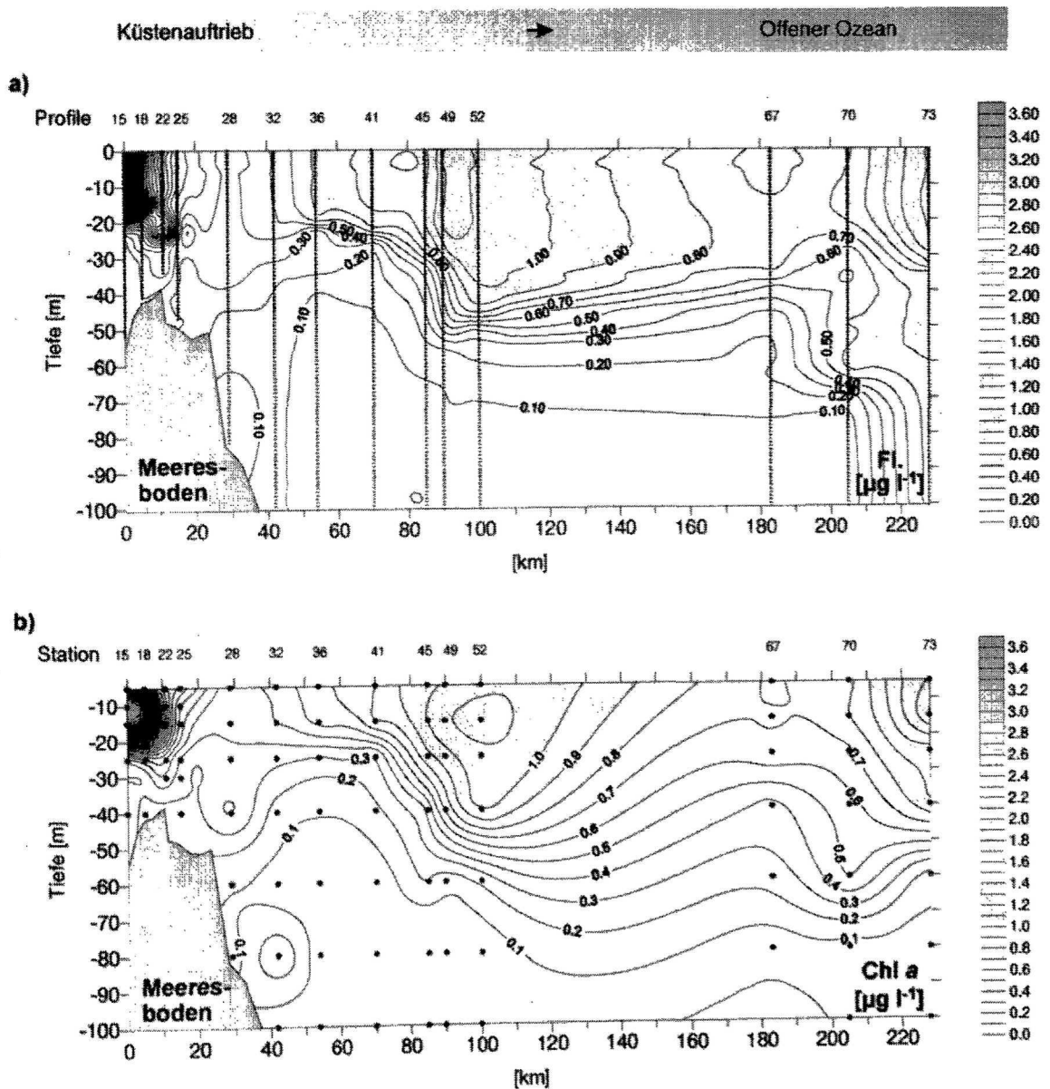
Abb. 5.6a+b In situ Chl a -Fluoreszenz (a) und fluorometrisch ermittelte Chl a -Konzentration (b) jeweils in \mu\text{g l}^{-1} in den oberen 100 m der Wassersäule entlang der Drifttrajektorie während der Expedition SONNE 120.
