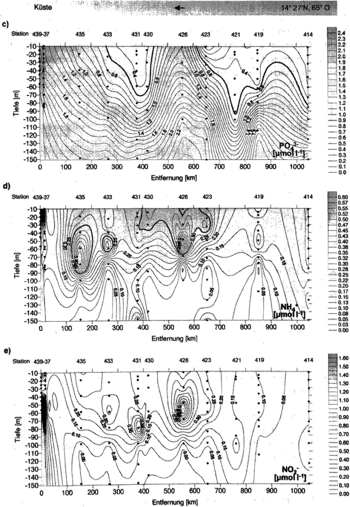
Abb. 4.17c-e Konzentrationen von c) Phosphat, d) Ammonium und e) Nitrit in \mu\text{mol l}^{-1} in den oberen 150 m der Wassersäule entlang des Schnittes von 14° 27'N, 65° O bis in den Küstenauftrieb vor Oman während der Expedition METEOR 32/5. Die 0.30 \mu\text{mol l}^{-1} Phosphat- und die 0.30 \mu\text{mol l}^{-1} Ammonium-Isoplethe ist jeweils fettgedruckt.
