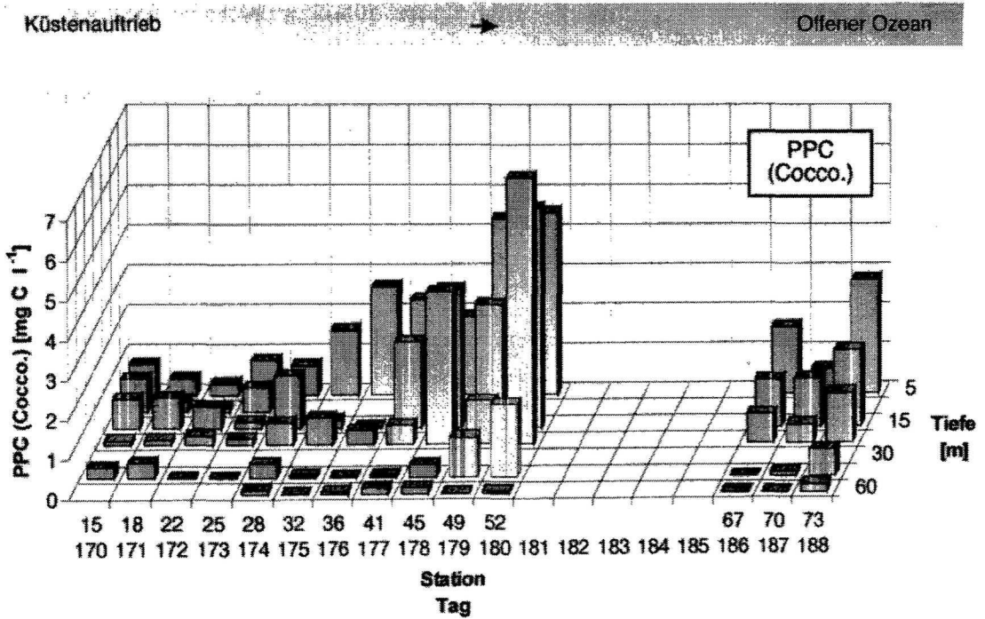
Abb. 5.18 Coccolithophoridenkohlenstoff (Cocco. PPC) in \text{mg l}^{-1} in verschiedenen Tiefen der euphotischen Zone entlang der Drifttrajektorie während der Expedition SONNE 120.
