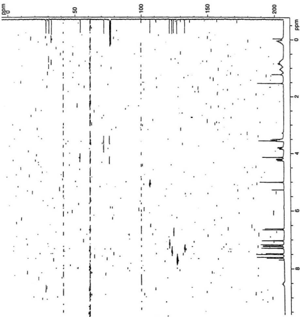
^1\text{H} - ^{13}\text{C} HETCORR
