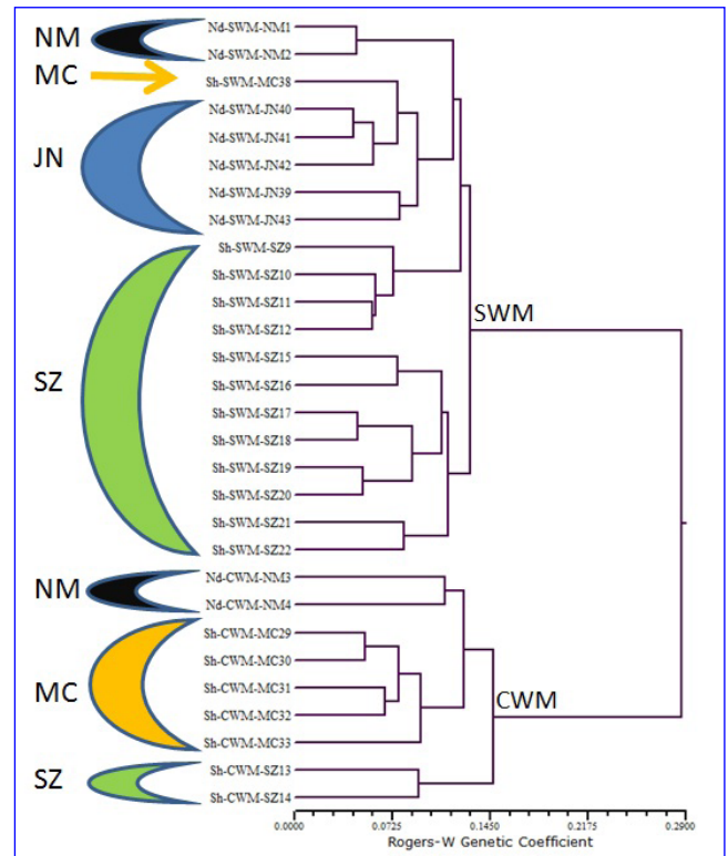
Fig. 7. DNA-markör baserat dendrogram, visar graden av likhet mellan olika lantraser, färgen anger vilken gård de kommer från, CWM cow-melon, SWM söt vattenmelon. Inom de två huvudgrupperna, SWM och CWM, är lantraser från samma gård mest lika varandra.
