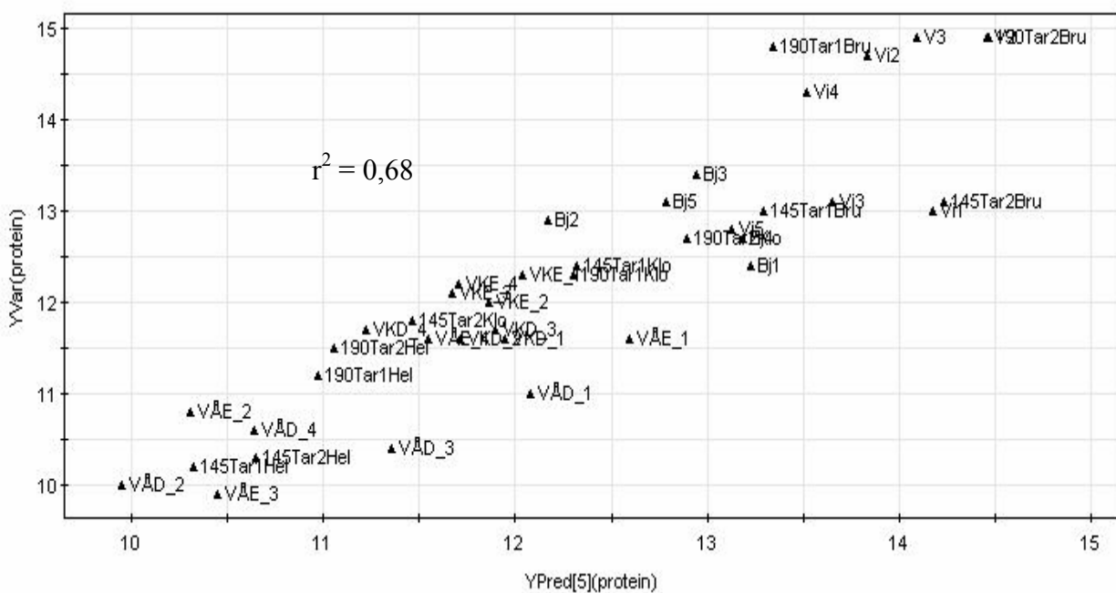
Figur 10. Prognos av proteinhalt i Tarso-ve. Korsvalidering med kombination av sensordata från 2000 och 2001, totalt 40 rutor varav 12 från 2000. Prognosvärden på x-axeln och uppmätta på y-axeln.
