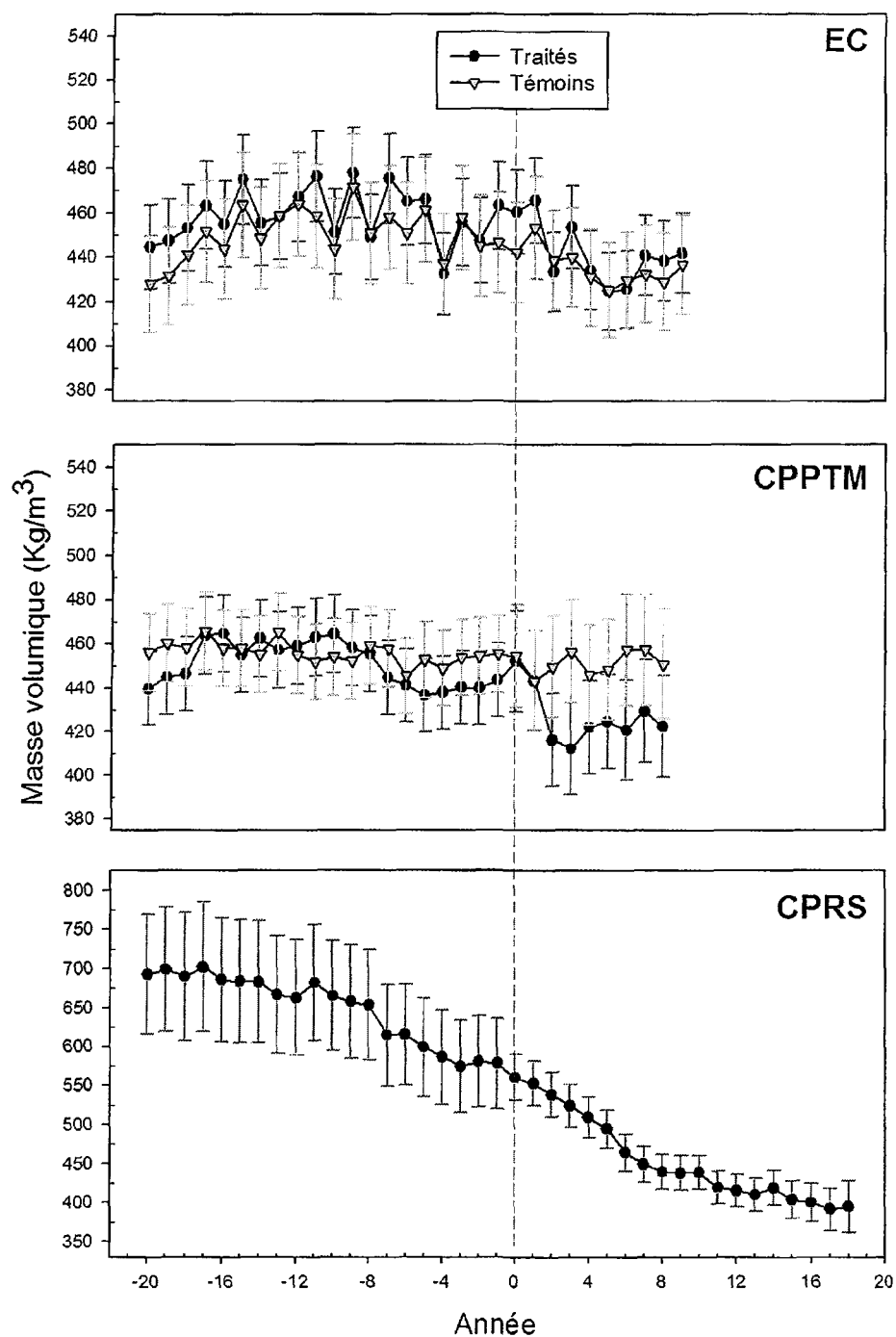
Figure 16. Courbes moyennes de la masse volumique annuelle (Kg/m 3 ) avec les intervalles de confiance, par intervention, comparées avec les stations témoins. La ligne pointillée représente l'année de l'intervention. Les astérisques (*) représentent les résultats significatifs du test de comparaisons multiples par tranche.
