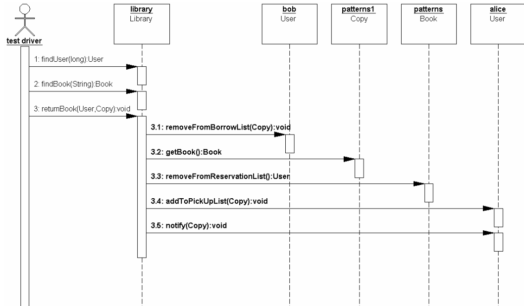
Abbildung 2: UML Sequenzdiagramm
