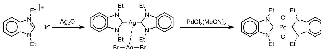
Schema 2: Sintesi di un complesso dicarbenico mononucleare di Pd(II) per transmetallazione da un complesso dicarbenico di Ag(I) [4] .
