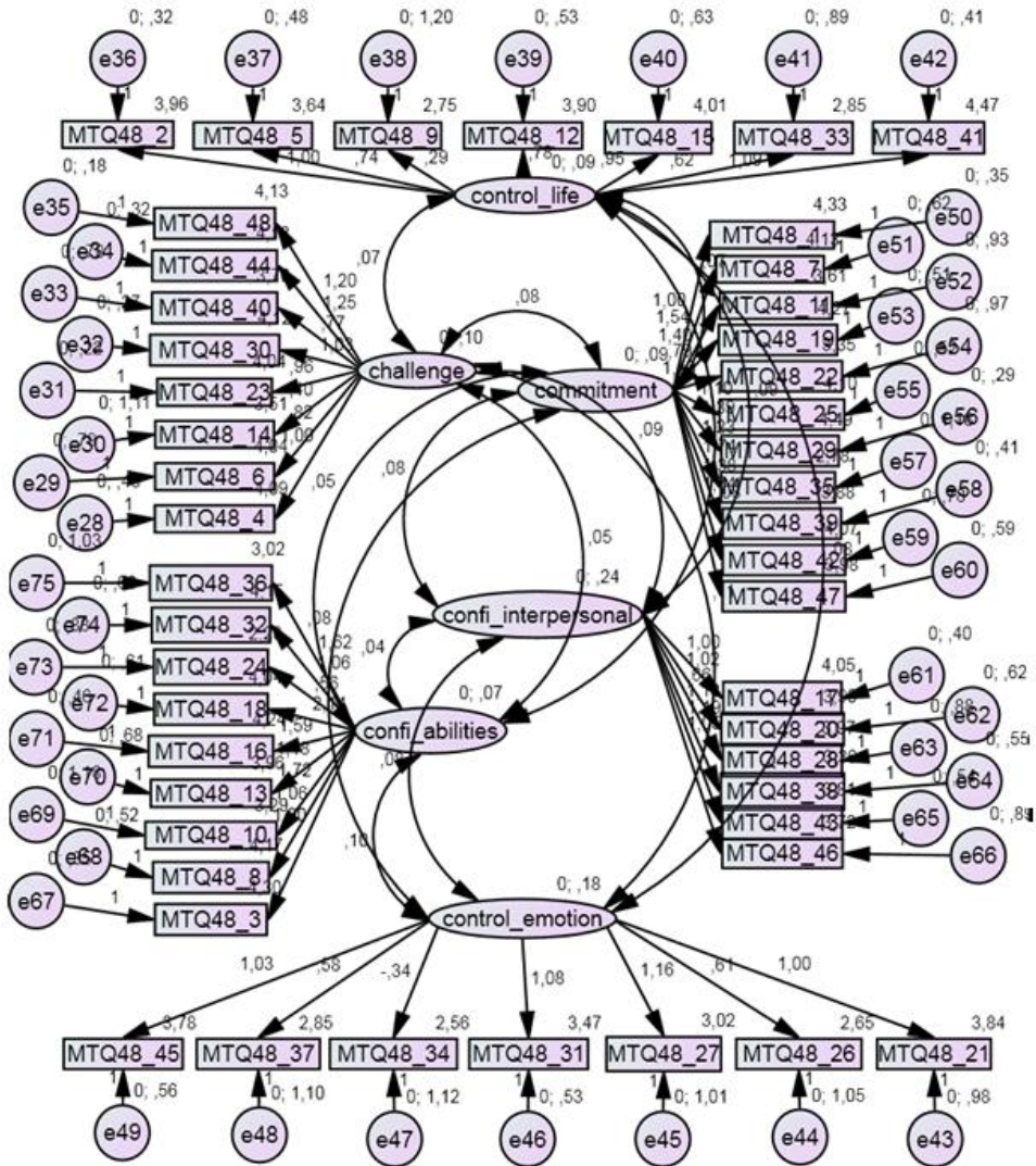
Abb. 8 Theoretische Faktorenstruktur des MTQ48
