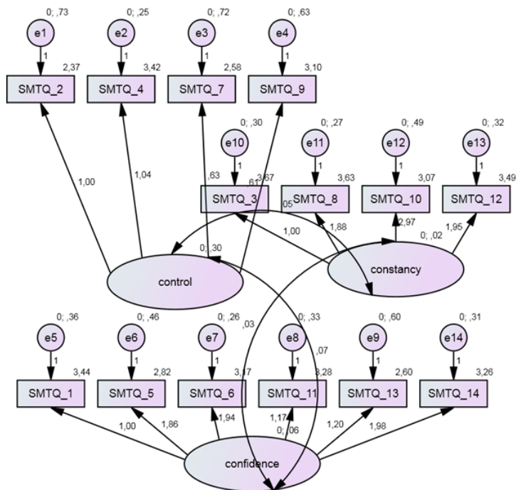
Abb. 9 Theoretische Faktorenstruktur des SMTQ
