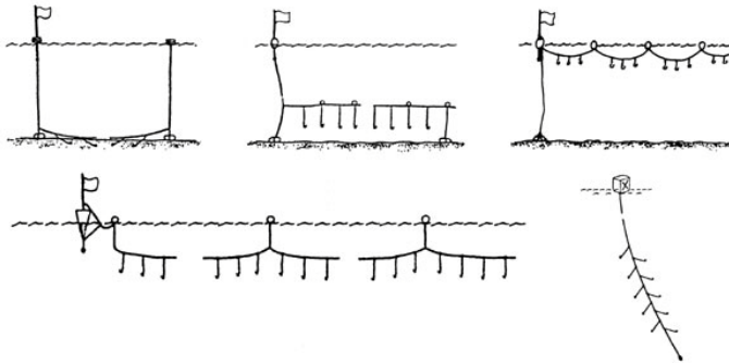
Abb. 11: Haken und Leinen (FAO, 2012a)
