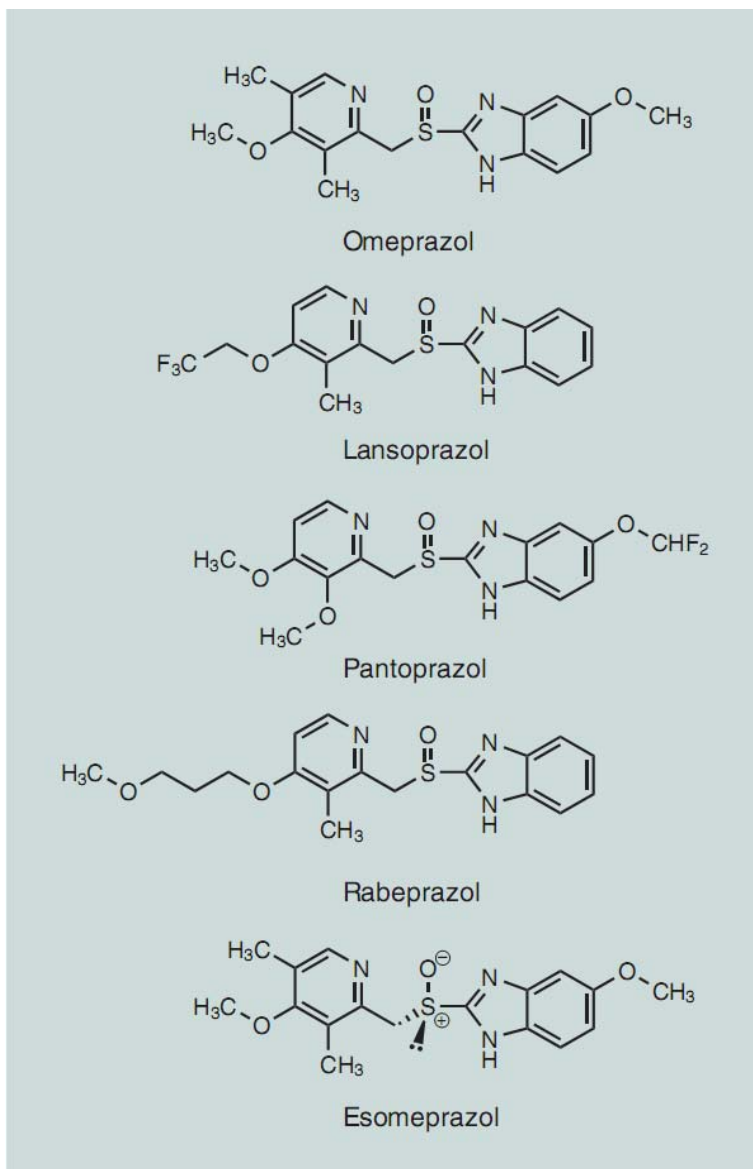
Abbildung 1 Chemische Struktur der PPIs (Schubert-Zsilavec und Stark, 2005)
