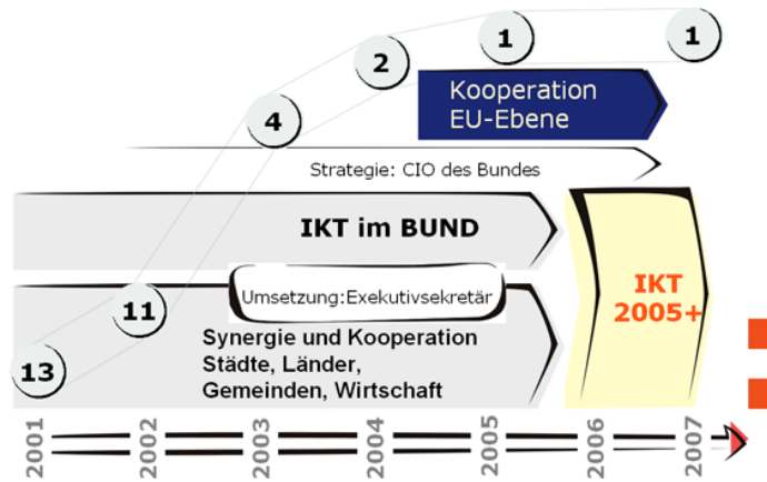
Abb. 10: E-Government-Strategie 2005+
