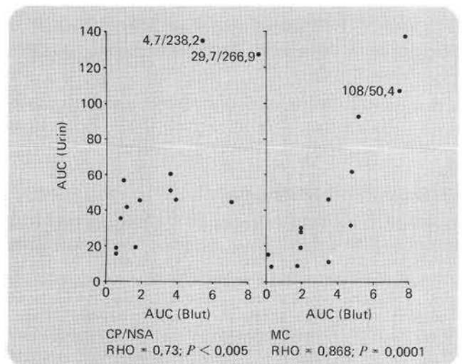
Abb. 3. Korrelation der ^{51}\text{Cr} -EDTA-Urinausscheidung mit der ^{51}\text{Cr} -EDTA-Aktivität im Blut, ausgedrückt als AUC. CP/NSA = Patienten mit chronischer Polyarthrits unter NSA, MC = Patienten mit Morbus Crohn. RHO = Rang-Korrelationskoeffizient nach Spearman.
