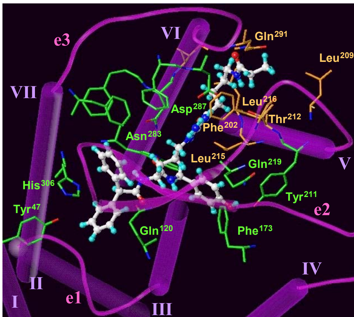
Abbildung 4-3: Mögliche Bindung von 82 an den humanen Y_1 -Rezeptor auf Basis des Modells für BIBP 3226 [Dove, 2002]. Die für die Wechselwirkung mit BIBP 3226 entscheidenden Aminosäuren sind grün, Aminosäuren, die zusätzliche Wechselwirkungen mit 82 eingehen können, sind orange eingefärbt.
