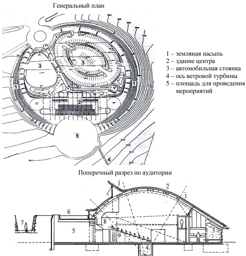
Рис.3 – Проект реновации энергетического центра в Делаболи, Корнвелл, Англия (архитекторы: Эдвард Куллинан & Architects):
