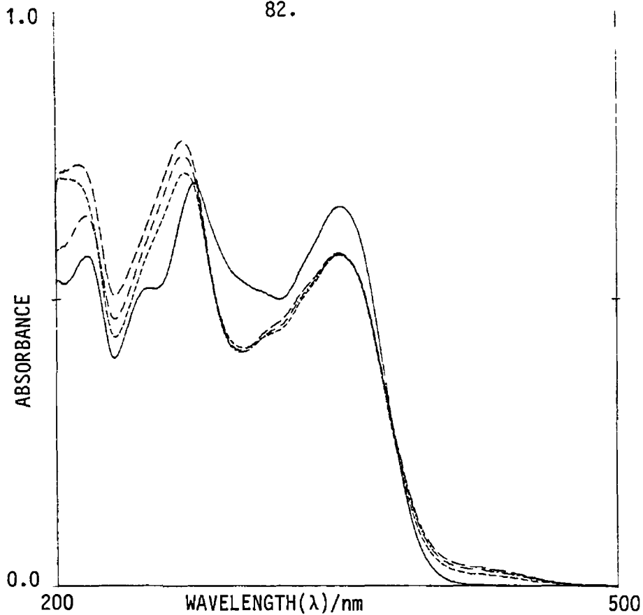
Fig. 21a Ultraviolet Spectra of Oxytetracycline hydrochloride (OTC) (—), OTC Fe(II) 1 1 (----), OTC Fe(II) 1 2 (-.-.-)
