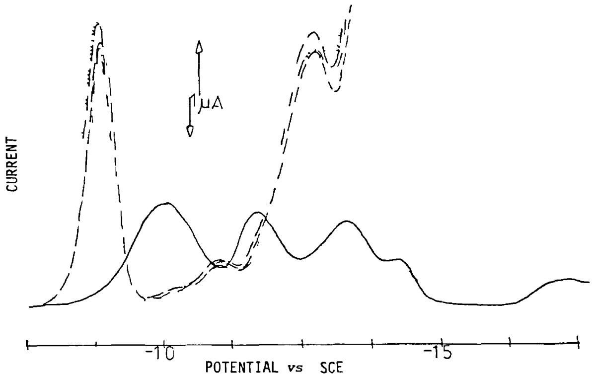
Fig 28b Differential Pulse Polarograms of OTC (—), OTC Fe(II) 1:5 (----), OTC Fe(II) 1:6 (- · - · -), OTC Fe(II) 1:7 (· · · · ·) and OTC Fe(II) 1:8 (— · — · —) in 0.1M KCl
