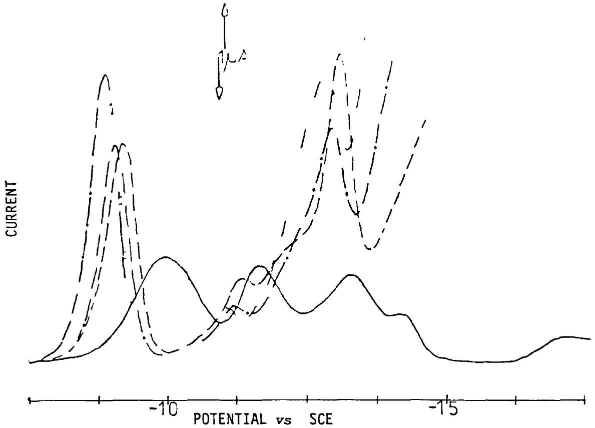
Fig. 28a Differential Pulse Polarograms of Oxytetracycline hydrochloride (OTC) (—), OTC Fe(II) 1:1 (----), OTC Fe(II) 1:2 (- · - · -), OTC Fe(II) 1:3 (· · · · ·), and OTC Fe(II) 1:4 (— · — · —) in 0.1M KCl
