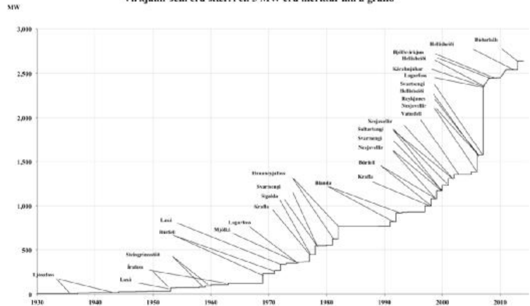
Virkjanasaga frá 1930 til 2014 Virkjanir sem eru stærri en 5 MW eru merktar inn á grafið
