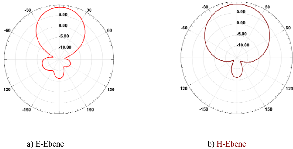
Bild 6.15 Die Darstellung der Directivity in E-Ebene und H-Ebene bei 435 MHz
