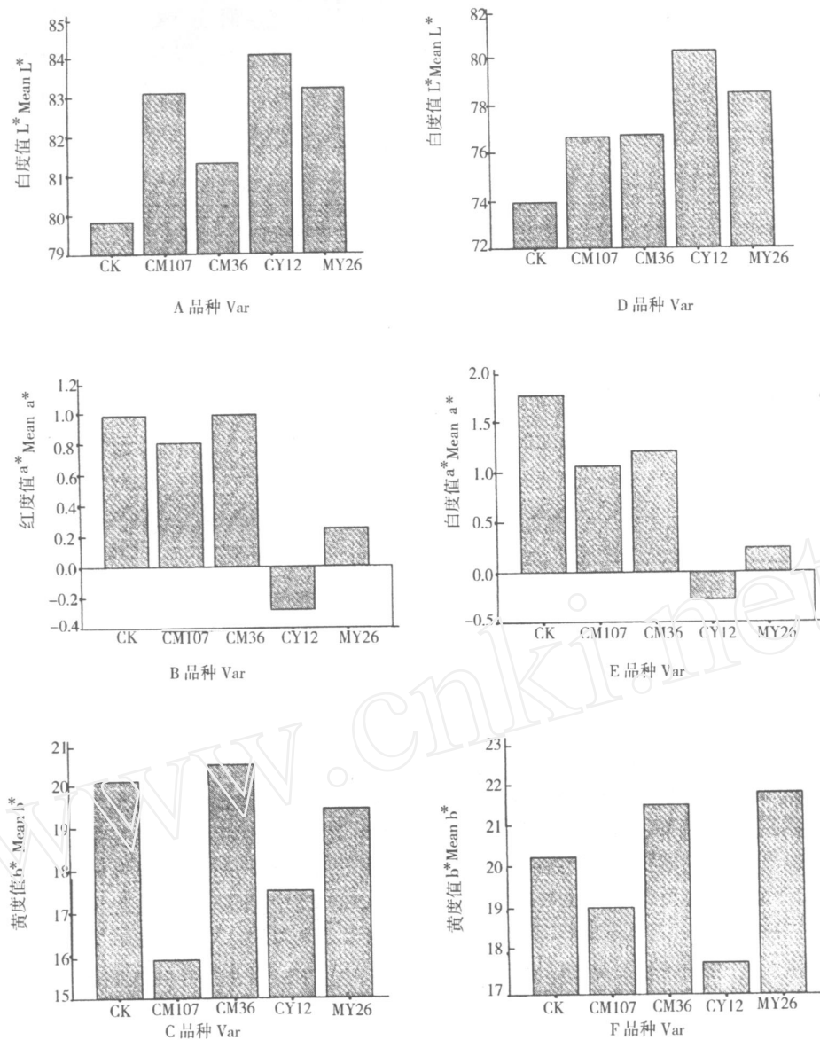
图1 面条颜色(L * 、a * 、b * ) 在 0 h(A~C)、24 h(D~E) 的表现
