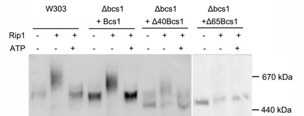
Abb. 3.23: Wechselwirkung von BCS1-Varianten mit Rip1
