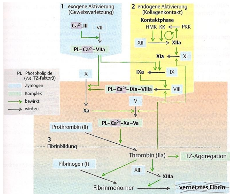
Abbildung 2.2: Gerinnungssystem [37]
