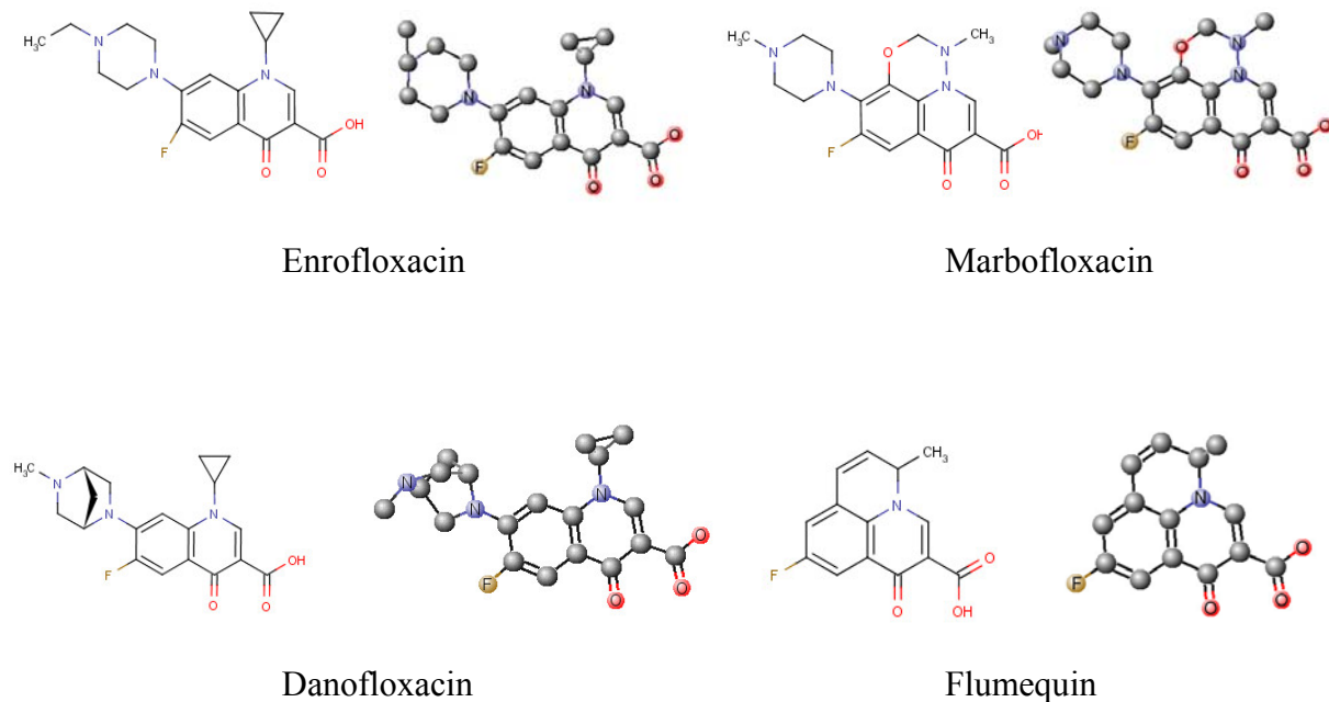
Abbildung 4: Strukturformeln von Fluorchinolonen, die für Rinder, von denen Milch für den menschlichen Verzehr gewonnen wird, zugelassen sind
