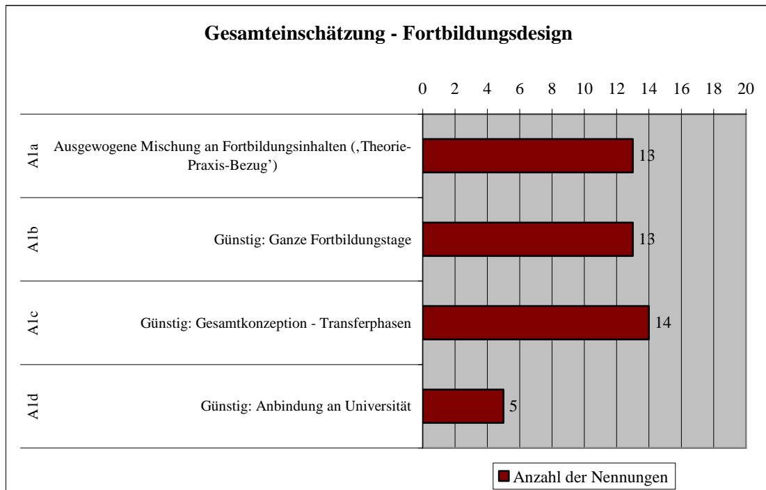
Abb. 12: Gesamteinschätzung - Fortbildungsdesign
