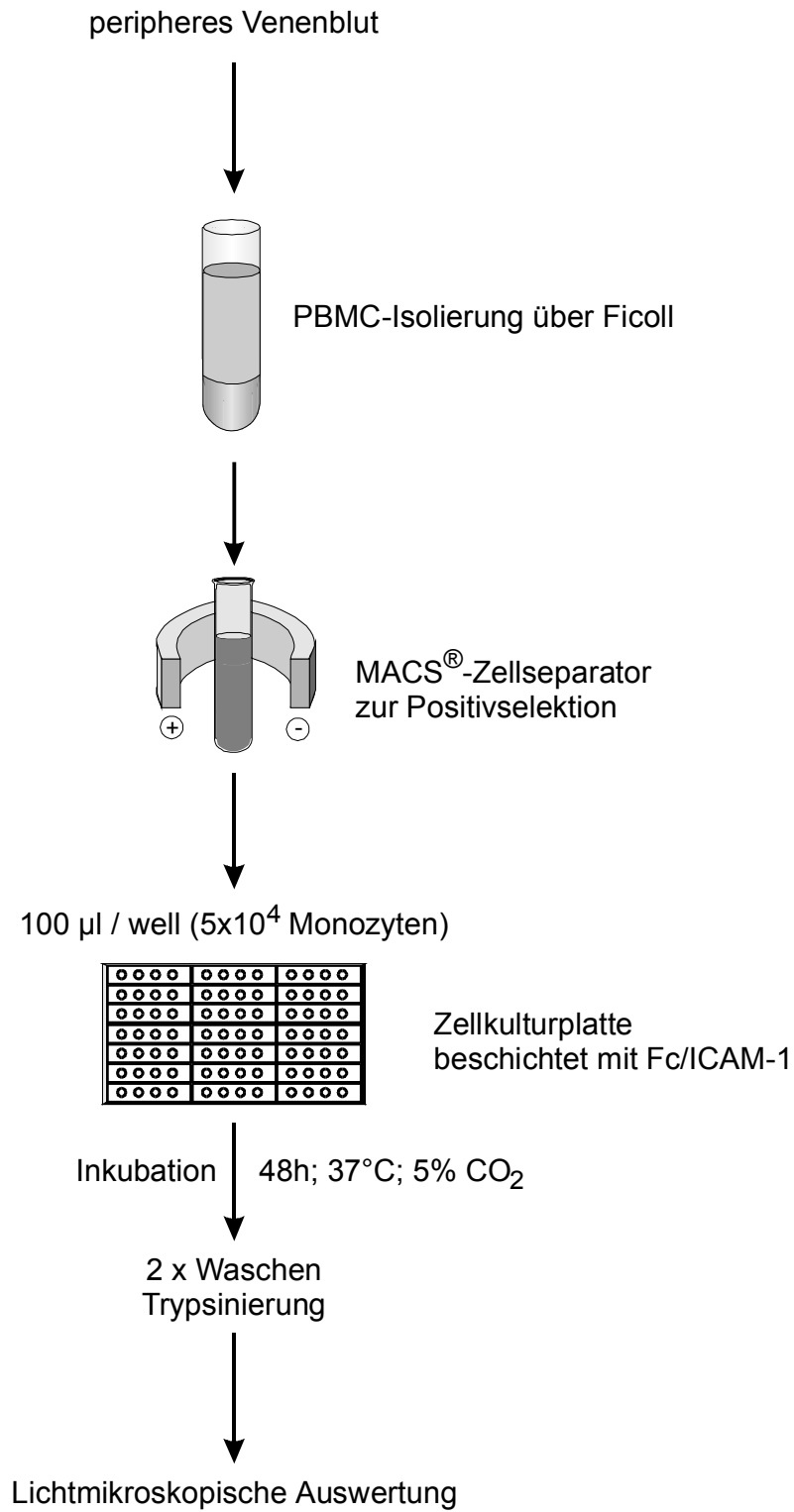
Abbildung 2-6: Adhäsionsassay
