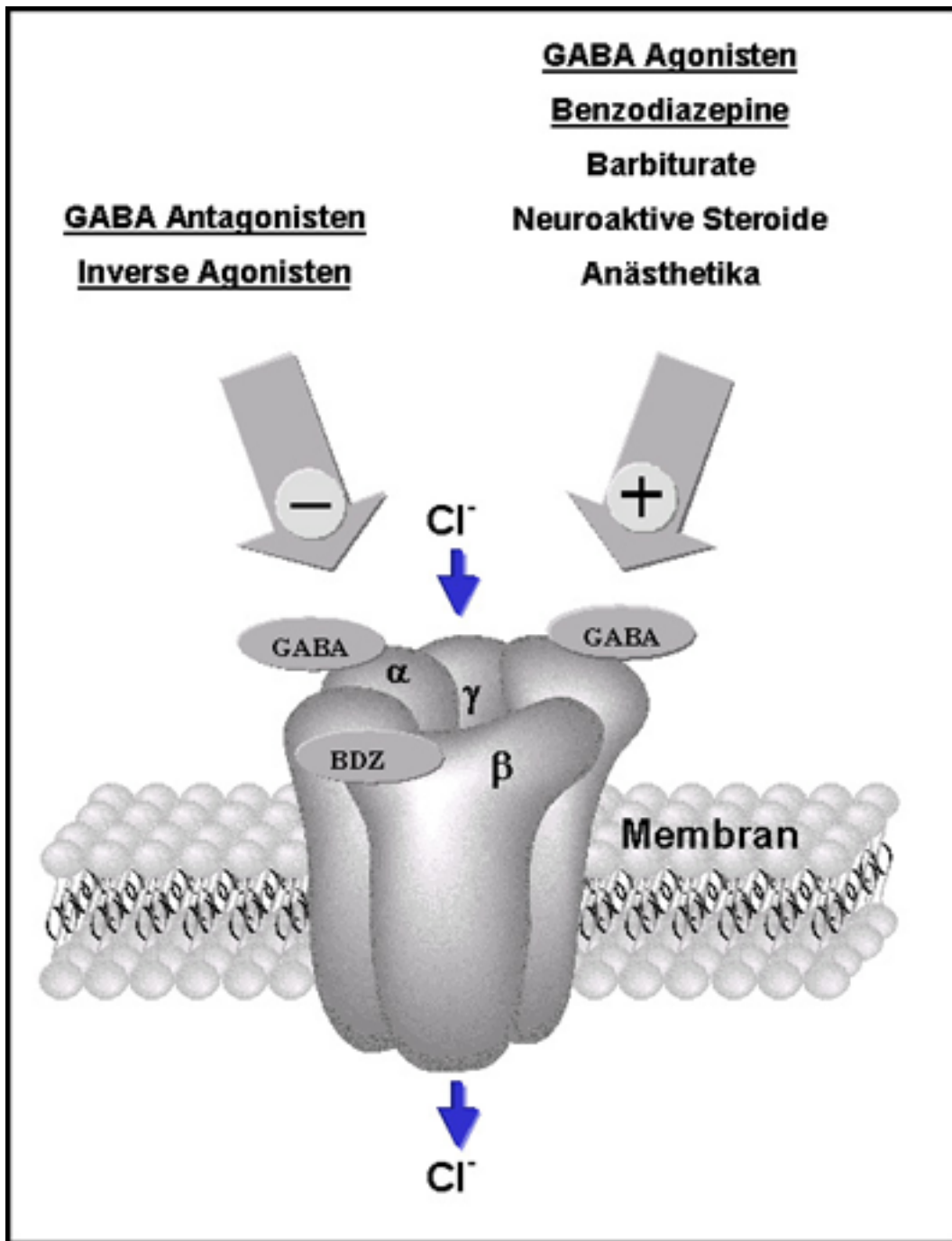
Abb. 3: GABA-Benzodiazepinrezeptorkomplex
