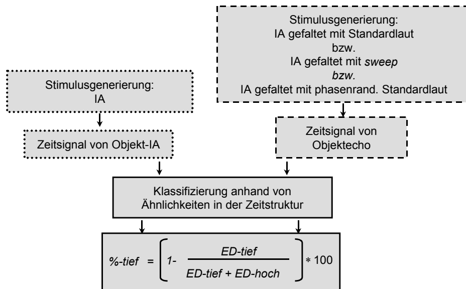
Abbildung 11: Schematische Darstellung von Modell 1 (gepunktete Linien) und Modell 2 (gestrichelte Linien). Beide Modelle beruhen auf dem gleichen Klassifizierungsparadigma (durchgezogene Linien). Das Eingangssignal für Modell 1 ist das Zeitsignal der Objekt-IAs; das Eingangssignal für Modell 2 ist das Zeitsignal der Objektechos. Anhand der EDs der einzelnen zu testenden Eingangssignale (IA1-10 bzw. Echo1-10) zu den gemittelten tieffrequenten (ED-tief) und den gemittelten hochfrequenten Eingangssignalen (ED-hoch) konnte die Klassifizierung des Eingangssignals als tieffrequent (%tief) simuliert werden.
