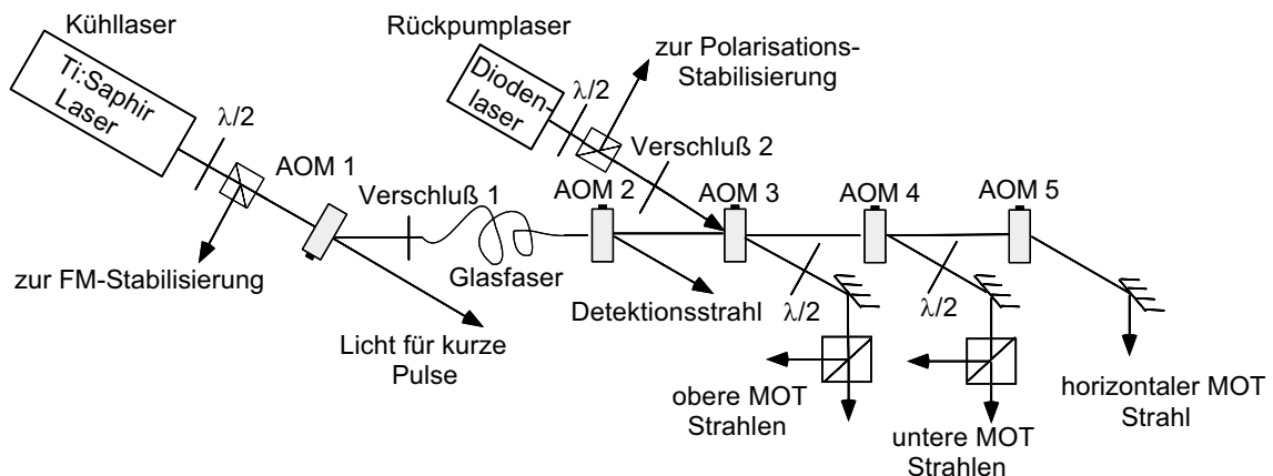
Abb. 5.9: Schematischer Überblick über den optischen Aufbau. Neben dem Ti:Saphir Laser und dem Diodenlaser sind die wichtigsten optischen Elemente gezeigt, deren Bedeutung und Funktionsweise im Text erklärt wird.
