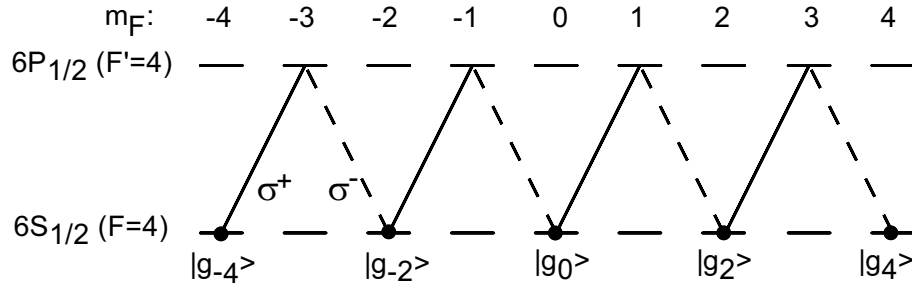
Abb. 3.1: Niveauschema für einen geschwindigkeitsunabhängigen Dunkelzustand für den 6S_{1/2}(F=4) \rightarrow 6P_{1/2}(F'=4) Übergang der Cäsium D1-Linie. Wird das Atom gleichzeitig mit \sigma^+ - und \sigma^- -polarisiertem Licht der gleichen Ausbreitungsrichtung beleuchtet, so existiert ein Dunkelzustand in F=4 , der aus den fünf geradzahigen m_F -Niveaus besteht.
