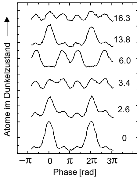
Abb. 3.8: Experimentelle Interferenzsignale für den Dunkelzustand in F = 3 als Funktion der Phase des zweiten Ramsey-Pulses. Die einzelnen Spektren entsprechen wiederum den in \text{mW/cm}^2 angegebenen Intensitäten I_{TP} .
