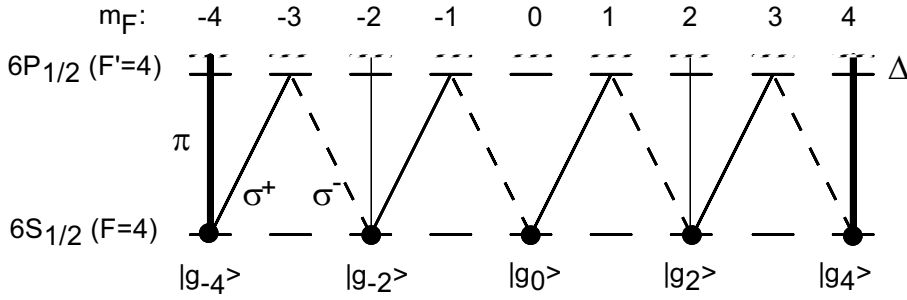
Abb. 3.3: Relevante Energieniveaus von Cäsium. Die Matrixelemente für das \pi -polarisierte Licht sind proportional zu m_F (verdeutlicht durch die verschiedenen Strichstärken).
