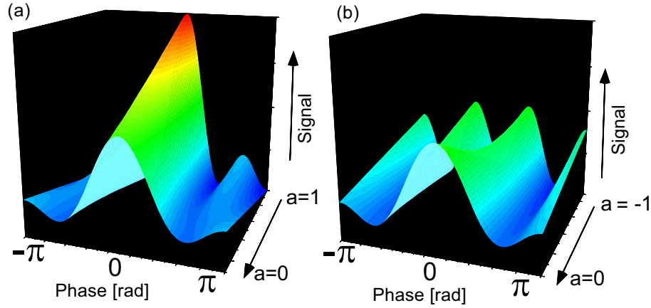
Abb. 4.2: Theoretisches Interferenzsignal eines Vierstrahl-Interferometers (a) mit konstanter Phasendifferenz zwischen benachbarten Pfaden und (b) mit einer zusätzlichen Phase von \pi in einem der äußeren Pfade. Aufgetragen ist die Anzahl der Atome im Dunkelzustand sowohl als Funktion der Phase des zweiten Ramsey-Pulses als auch der Kopplungsstärke an die Umgebung. Um Übereinstimmung mit dem Experiment zu gewährleisten, wurden die Interferenzsignale unter der Annahme berechnet, daß die interferierenden Wahrscheinlichkeitsamplituden der zwei äußeren Pfade um einen Faktor 5/3 höher als die Amplituden der zwei inneren Pfade sind.
