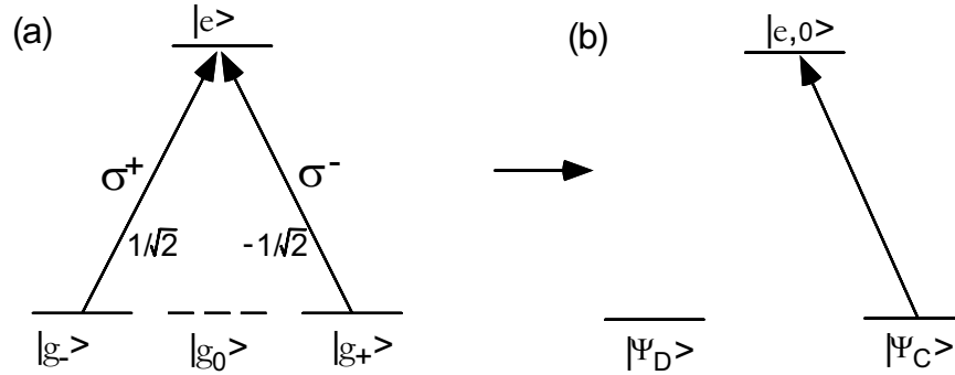
Abb. 2.3: Schematische Darstellung des Übergangs von den Eigenfunktionen |g_{\mp}\rangle zu den neuen Eigenfunktionen |\Psi_D\rangle und |\Psi_C\rangle . (a) Erlaubte Übergänge mit entsprechenden Clebsch-Gordan Koeffizienten. Da der Übergang |e\rangle \leftrightarrow |g_0\rangle verboten ist, werden alle Atome innerhalb weniger Fluoreszenzzyklen in die Zustände |g_{-}\rangle und |g_{+}\rangle gepumpt. (b) Die durch eine Basistransformation resultierenden neuen Eigenzustände |\Psi_D\rangle und |\Psi_C\rangle . Der Zustand |\Psi_D\rangle koppelt nicht mehr an das Lichtfeld.
