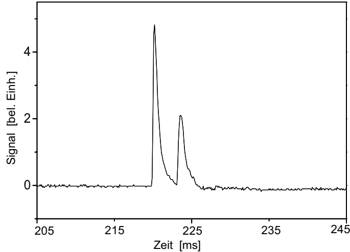
Abb. 5.14: Flugzeitspektrum aufgenommen mit der frequenzmodulierten Fluoreszenzmethode. Das Spektrum hat ein Signal-zu-Rausch-Verhältnis von größer als 250 und einen vernachlässigbaren Untergrund (der Beitrag des thermischen Hintergrundgases liegt unterhalb der Detektionsgrenze).
