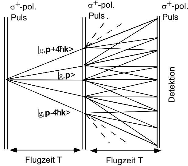
Abb. 5.2: Raum-Zeit-Darstellung des Vielstrahl-Atominterferometers basierend auf einer Sequenz dreier kurzer Lichtpulse. Dabei unterscheiden sich benachbarte Teilstrahlen im Impuls um 2\hbar\mathbf{k} . Nur die Trajektorien, die zu einem geschlossenen Interferometer gehören, sind gezeigt. Während des dritten Lichtpulses kreuzen sich mehrere Pfade. Dabei interferieren die Atome in verschiedenen Familien von Wellenpaketen.
