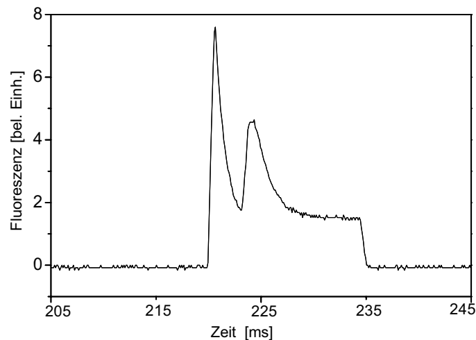
Abb. 5.12: Flugzeitspektrum mit gepulstem Detektionsstrahl. Aufgetragen ist die Fluoreszenz als Funktion der Zeit. Der Detektionsstrahl wird zu der Zeit angepulst, bei der die maximale Zahl an Atomen durch den Detektionsbereich fliegt ( t = 220 \text{ ms} ). Die resultierende Fluoreszenz ergibt den ersten Peak. Das Rückpumplicht im Detektionsstrahl wird 4 \text{ ms} später angepulst. Dies ergibt den zweiten Peak.
