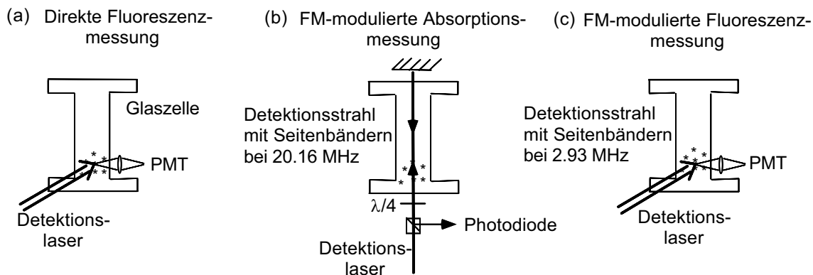
Abb. 5.10: Verwendete Methoden zur Detektion der ultrakalten Atome. (a) Direkte Fluoreszenzmessung, (b) frequenzmodulierte Absorptionsmessung und (c) frequenzmodulierte Fluoreszenzmessung. PMT steht für Photoelektronen-Vervielfacher.
