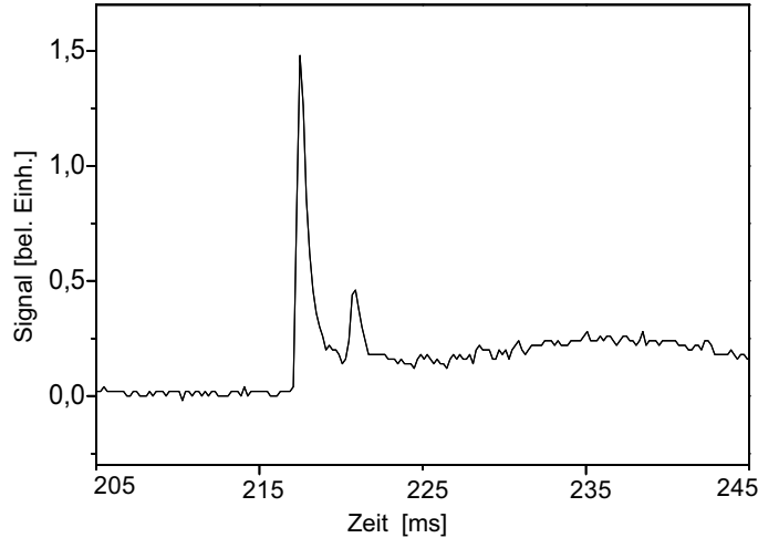
Abb. 5.13: Flugzeitspektrum aufgenommen mit der frequenzmodulierten Absorptionsmethode.
