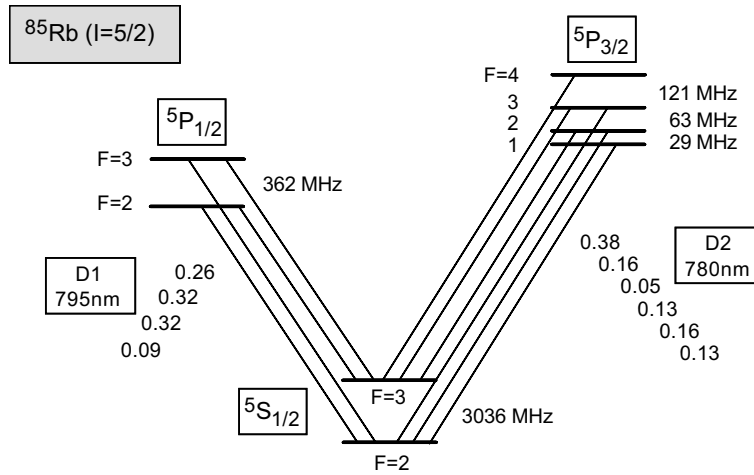
Abb. A.2: Linienstärken und Hyperfeinintervalle von ^{85}\text{Rb} . Angaben wie in Abb. A.1.
