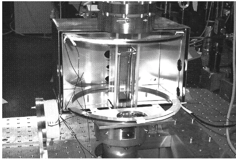
Abb. 5.8: Gezeigt ist ein Photo der Glaszelle, das während des Aufbaus des Systems aufgenommen wurde. In der Mitte ist die Glaszelle zu sehen, in der die Rubidiumatome gefangen, gekühlt, hochgeworfen und detektiert werden. Außerdem sind Teile der \mu -Metallabschirmung und ein Spulenpaar zur Kompensation der vertikalen Magnetfelder abgelichtet. Links neben der Apparatur sieht man eine der MOT-Spulen, die zum Zeitpunkt der Aufnahme noch nicht eingebaut waren.
