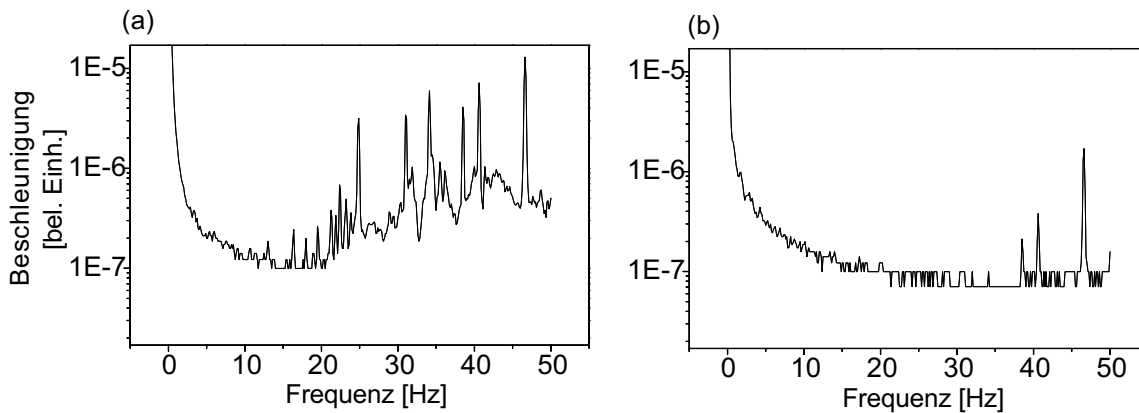
Abb. 5.5: Aufnahme des Vibrationsspektrums. Aufgetragen ist die Beschleunigung des Vibrationssensors über das zugehörige Frequenzspektrum. (a) Vibrationsspektrum des optischen Tisches, auf dem das Experiment aufgebaut ist. (b) Vibrationsspektrum des vibrationsisolierten Spiegels.
