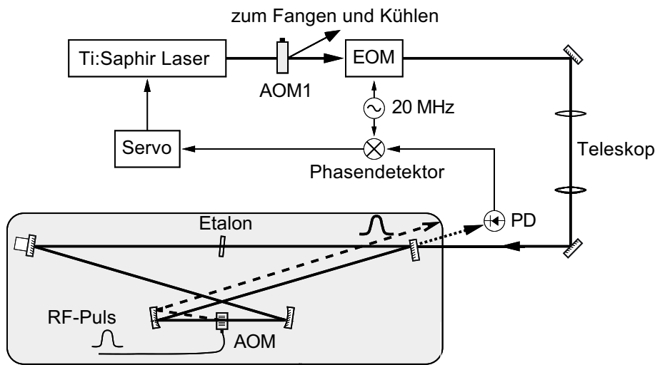
Abb. 5.3: Experimenteller Aufbau zur Erzeugung der Lichtpulse. Das in dem Resonator gespeicherte und überhöhte Licht wird mit einem schnellen akusto-optischen Modulator (AOM), der sich in einem der Foki des Resonators befindet, in einem kurzen Puls ausgekoppelt.
