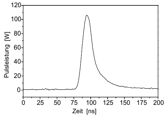
Abb. 5.4: Optischer Puls, der durch einen 20 ns langen Radiofrequenzpuls mit 10 W Radiofrequenzleistung erzeugt wurde. Der Resonator war für die Aufnahme auf eine Leistung von 235 W stabilisiert. Die Pulsform ist nicht symmetrisch, da die Abklingzeit der verwendeten Photodiode (Antel AR-S2) langsamer als die Anstiegszeit ist.
