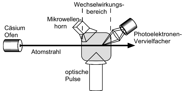
Abb. 4.3: Schematischer Überblick über den experimentellen Aufbau.
