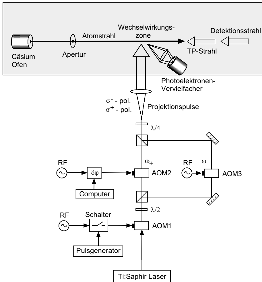
Abb. 3.5: Vereinfachte Darstellung des experimentellen Aufbaus des Vielstrahl-Ramsey-Experiments.
