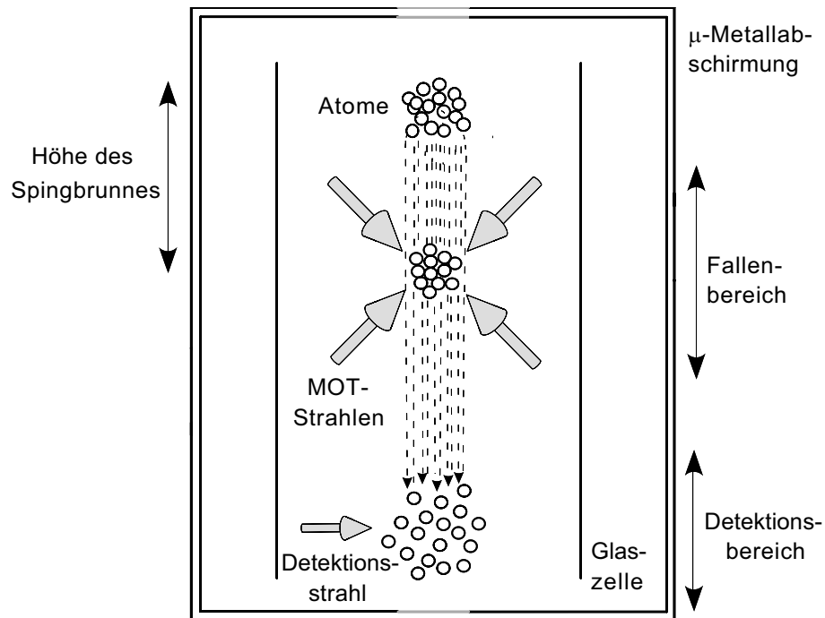
Abb. 5.6: Schematische Darstellung des atomaren Springbrunnens. Die Atome werden im Fallenbereich gefangen und gekühlt, dann hochgeworfen und schließlich sechs Zentimeter unterhalb der Fallenregion detektiert. Die ganze Anordnung befindet sich im Inneren einer zweilagigen Magnetfeldabschirmung aus \mu -Metall.
