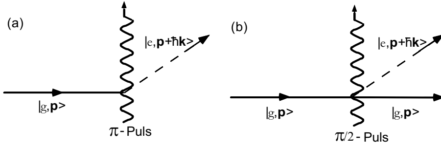
Abb. 2.1: Rückstoßdiagramm für die Wechselwirkung eines \pi - beziehungsweise \pi/2 -Pulses mit einem Zwei-Niveau-System. Die vertikale Achse entspricht der Position eines Atoms relativ zu einem Bezugssystem, das entlang der ursprünglichen Trajektorie des Atoms frei fällt. Die horizontale Achse beschreibt die Zeitentwicklung. (a) Ablenkung der Trajektorie durch einen \pi -Puls. (b) Kohärente Aufspaltung durch einen \pi/2 -Puls.
