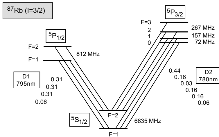
Abb. A.3: Linienstärken und Hyperfeinintervalle von ^{87}\text{Rb} . Angaben wie in Abb. A.1.
