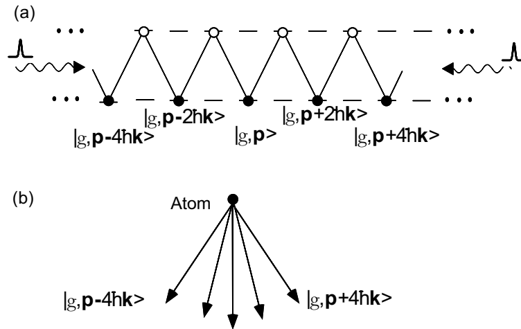
Abb. 5.1: Prinzip der atomaren Strahlteiler für ein Zwei-Niveau-System in einer resonanten, gepulsten Stehwelle. (a) Durch wiederholte Absorption und stimulierte Emission werden Komponenten mit unterschiedlichen Impulsen bevölkert. Die im angeregten Zustand befindlichen Komponenten zerfallen nach dem Puls spontan. Für einen offenen atomaren Übergang verbleiben nur die Komponenten im Grundzustand. (b) Räumliche Darstellung der erreichten kohärenten Aufspaltung.
