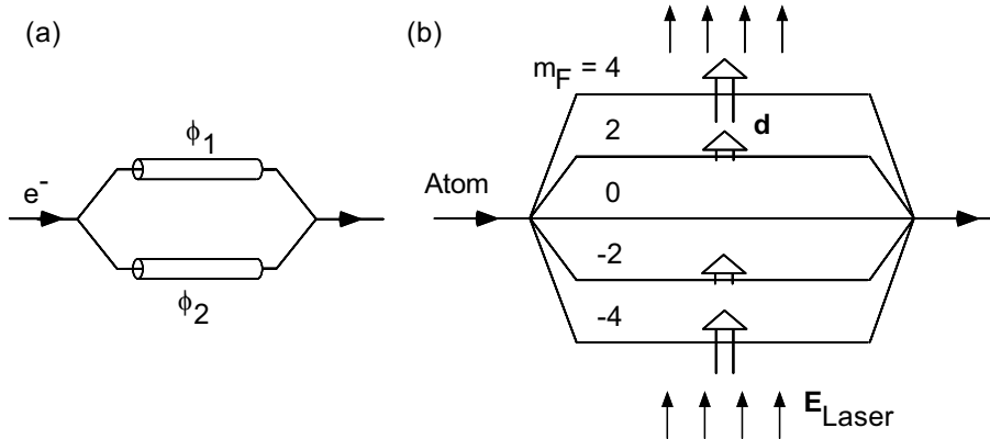
Abb. 3.2: Schematische Darstellung des elektrischen Aharonov-Bohm-Effektes (a) mit Elektronen und zwei interferierenden Teilstrahlen und (b) mit neutralen Atomen und fünf interferierenden Teilstrahlen. Man beachte die quadratische Abhängigkeit des induzierten Dipolmomentes \mathbf{d} von der magnetischen Quantenzahl m_F .
