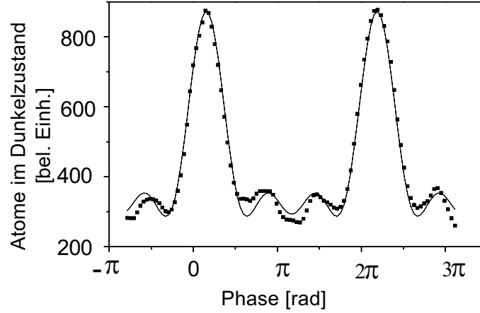
Abb. 4.6: Vierstrahl-Interferenzsignal für den Dunkelzustand in F = 3 als Funktion der Phase des zweiten Ramsey-Pulses. Das Spektrum wurde aufgenommen mit konstanter Phasendifferenz zwischen benachbarten Pfaden. An die experimentellen Werte wurde ein theoretisches Modell angepaßt, das die Gewichte der einzelnen Beiträge zur Interferenz berücksichtigt (durchgezogene Linie). Die Hauptmaxima sind leicht von Phase 0 und 2\pi verschoben, da die Frequenzdifferenz der Ramsey-Pulse nicht exakt mit der Differenz zwischen den Zeeman-Unterniveaus übereinstimmt.
