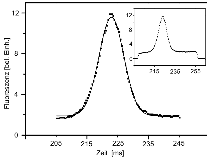
Abb. 5.11: Flugzeitspektrum zur Temperaturbestimmung der kalten Atome. Aufgetragen ist die Fluoreszenz als Funktion der Zeit. An die Datenpunkte wurde eine Gaußverteilung angepaßt. Über die Breite dieser Verteilung ergibt sich eine Temperatur von 15.99 \pm 0.02 \mu\text{K} . Die kleine Abbildung zeigt das Spektrum über die volle Zeit des Detektionslaserpulses. Deutlich ist der durch Anregung des Rubidium-Hintergrundgases verursachte Untergrund zu erkennen.
