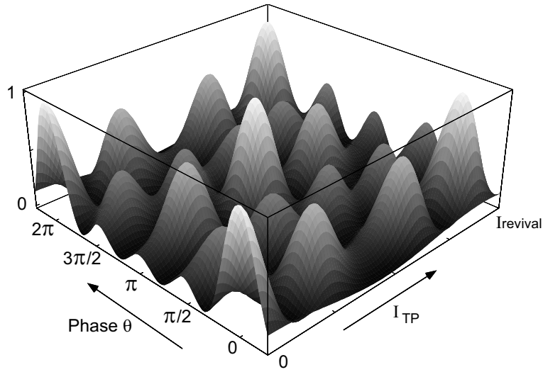
Abb. 3.4: Theoretisches Interferenzsignal für einen F = 4 nach F' = 4 Übergang als Funktion sowohl der Phase des zweiten Ramsey-Pulses \theta als auch der Intensität I_{TP} des Tensorpolarisationsstrahls. Entlang der vertikalen Achse ist das Verhältnis |\langle \Psi_D(T) | \Psi_D(0) \rangle|^2 der Atome im Dunkelzustand nach den zwei Pulsen zu den Atomen aufgetragen, die sich nach dem ersten Puls in diesem Zustand befanden.
