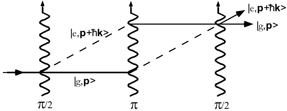
Abb. 2.2: Rückstoßdiagramm für eine \pi/2 - \pi - \pi/2 Pulssequenz. Mit dieser Sequenz ist das konzeptionell einfachste geschlossene Interferometer realisierbar.
