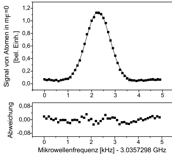
Abb. 5.15: Mikrowellenspektrum zur Überprüfung der Schuß-zu-Schuß-Fluktuationen der frequenzmodulierten Fluoreszenzmessung. Aufgetragen ist das Signal der im Zustand ( F = 3, m_F = 0 ) nachgewiesenen Atome als Funktion der Mikrowellenfrequenz. An die experimentellen Daten wurde eine Gaußverteilung angepaßt. Die Abweichungen der experimentellen Daten hiervon sind separat dargestellt. Daraus berechnen sich Schuß-zu-Schuß-Fluktuationen von 2%.
