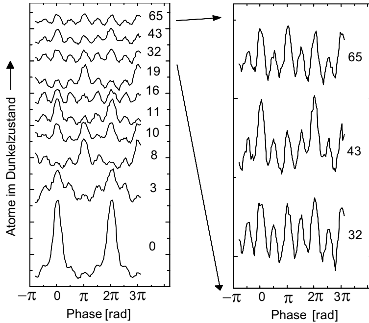
Abb. 3.7: Experimentelle Interferenzsignale für den Dunkelzustand in F = 4 als Funktion der Phase des zweiten Ramsey-Pulses. Die einzelnen Spektren entsprechen den am rechten Rand angegebenen Intensitäten I_{TP} in \text{mW}/\text{cm}^2 . Die drei Spektren mit den höchsten Intensitäten sind zusätzlich auf der rechten Seite in vergrößertem Maßstab gezeigt.
