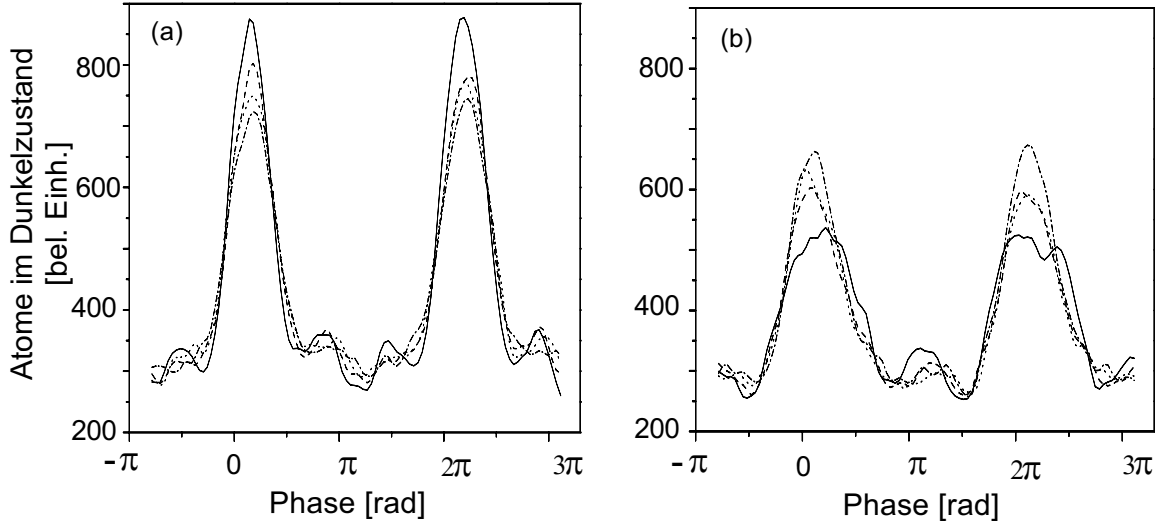
Abb. 4.7: Experimentelle Vielstrahl-Interferenzsignale als Funktion der Phase des zweiten Ramsey-Pulses. Die unterschiedlichen Spektren entsprechen unterschiedlichen Längen des optischen Pulses P_{\text{Decoh}} : ohne optischen Puls (durchgezogen), mit einem 4 \mu\text{s} langen optischen Puls (gestrichelt), mit einem 6 \mu\text{s} langen optischen Puls (gepunktet) und mit einem 9 \mu\text{s} langen optischen Puls (strichgepunktet). (a) Spektrum gemessen mit konstanter Phasendifferenz zwischen benachbarten Pfaden. Der Kontrast des Interferenzsignals nimmt mit zunehmender Pulsdauer ab. (b) Zusätzlich ist ein Phasenschub von \pi für m_F = 3 angelegt. Die Spektren sind für dieselben Wechselwirkungszeiten gezeigt. Wie man klar erkennt, nimmt hier der Kontrast mit zunehmender Pulsdauer zu.
