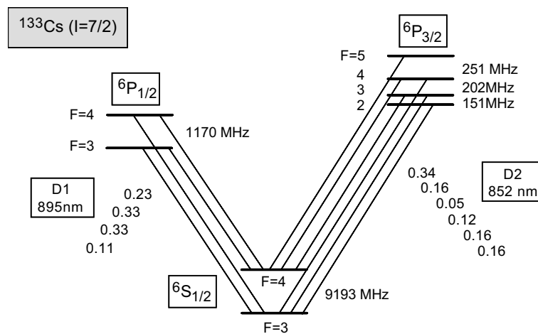
Abb. A.1: Linienstärken und Hyperfeinintervalle von Cäsium. Die Linienstärken sind jeweils auf Eins normiert. Die Hyperfeinintervalle wurden [Ari77] entnommen.
