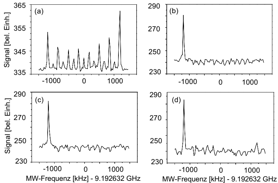
Abb. 4.5: Mikrowellenspektrum mit angelegtem Magnetfeld für verschiedene Leistungen I_{Dekoh} des Lasers zur Photonenstreuung. Aufgetragen ist das Fluoreszenzsignal von Atomen, die in das untere Hyperfeinniveau transferiert wurden als Funktion der angelegten Mikrowellenfrequenz. Aus den Spektren kann man die Besetzung der verschiedenen Zeeman-Unterniveaus des oberen F = 4 Hyperfeingrundzustandsniveaus ableiten. Die Spektren wurden aufgenommen mit (a) kein Rückpumplicht und kein Laser zur Photonenstreuung, (b) mit Rückpumplicht, (c) mit Rückpumplicht und I_{Dekoh} = 0.28 mW und (d) mit Rückpumplicht und mit I_{Dekoh} = 1.66 mW.
