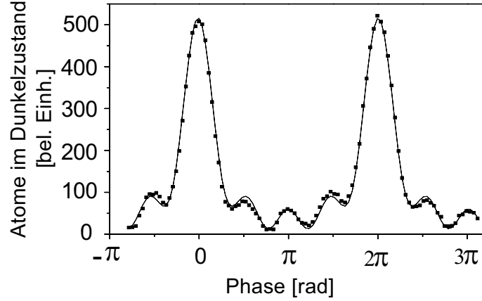
Abb. 3.6: Ramsey-Spektrum für den Dunkelzustand in F = 4 . Aufgetragen ist die Zahl der Atome im Dunkelzustand als Funktion der Phase des zweiten Ramsey-Pulses. An die experimentellen Werte wurde ein Fünfstrahl-Interferenzsignal angepaßt (durchgezogene Linie).
