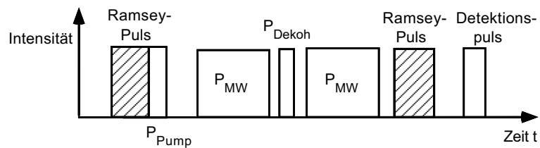
Abb. 4.4: Zeitlicher Ablauf des Experiments. Der optische Puls zur selektiven Photonenstreuung P_{Dekoh} wird zeitlich zwischen den zwei Mikrowellenpulsen eingestrahlt. Diese wiederum befinden sich zwischen den zwei Ramsey-Pulsen.
