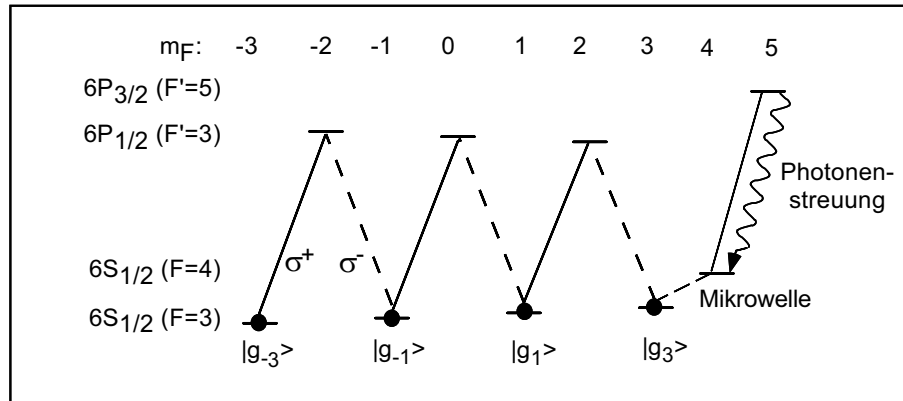
Abb. 4.1: Schematische Darstellung der relevanten Energieniveaus von atomarem Cäsium. Der Dunkelzustand besteht aus einer Überlagerung der ungeraden m_F -Niveaus des F = 3 Zustandes. Die |g_3\rangle -Komponente dieses Dunkelzustandes wird mit einem Mikrowellenpuls in den oberen Hyperfeinzustand transferiert. An diesem werden selektiv Photonen gestreut.
