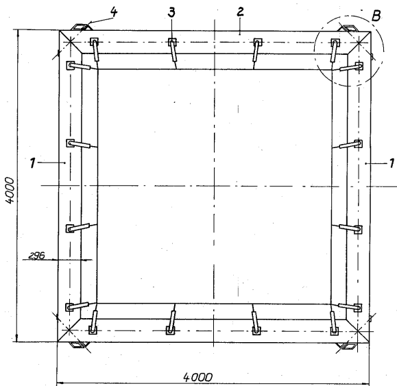
Abb. 2 : Aufbau des IOR- Pontonrahmens in der Draufsicht
