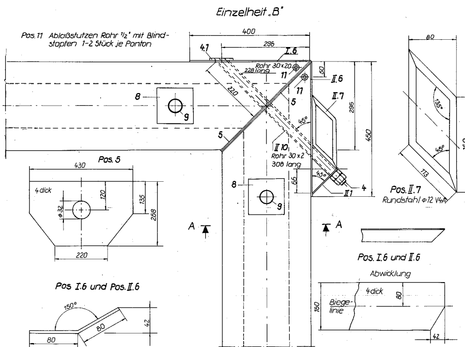
Abb. 2 : Aufbau des IOR- Pontonrahmens in der Draufsicht
