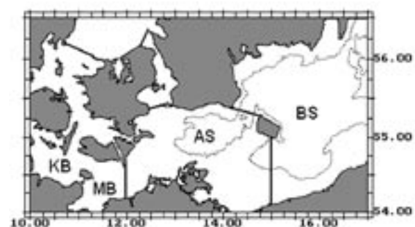
Abbildung 1: Untersuchungsgebiet mit Bezeichnung der verschiedenen Seegebiete (KB = Kieler Bucht, ICES-Gebiet 22; MB = Mecklenburger Bucht, ICES-Gebiet 22; AS = Arkonasee, ICES-Gebiet 24; BS = Bornholmsee, ICES-Gebiet 25).
