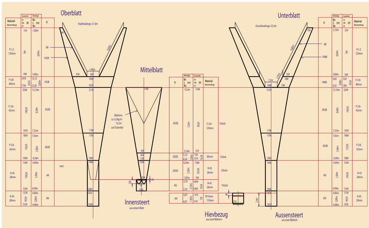
Abbildung 3: Maßstäbliche Fertigungszeichnung des Aalselektionstrawls Version 4. (Zeichnung: Rehme) Figure 3: To scale construction drawing of the eel selection trawl version 4. (Drawing: Rehme)
