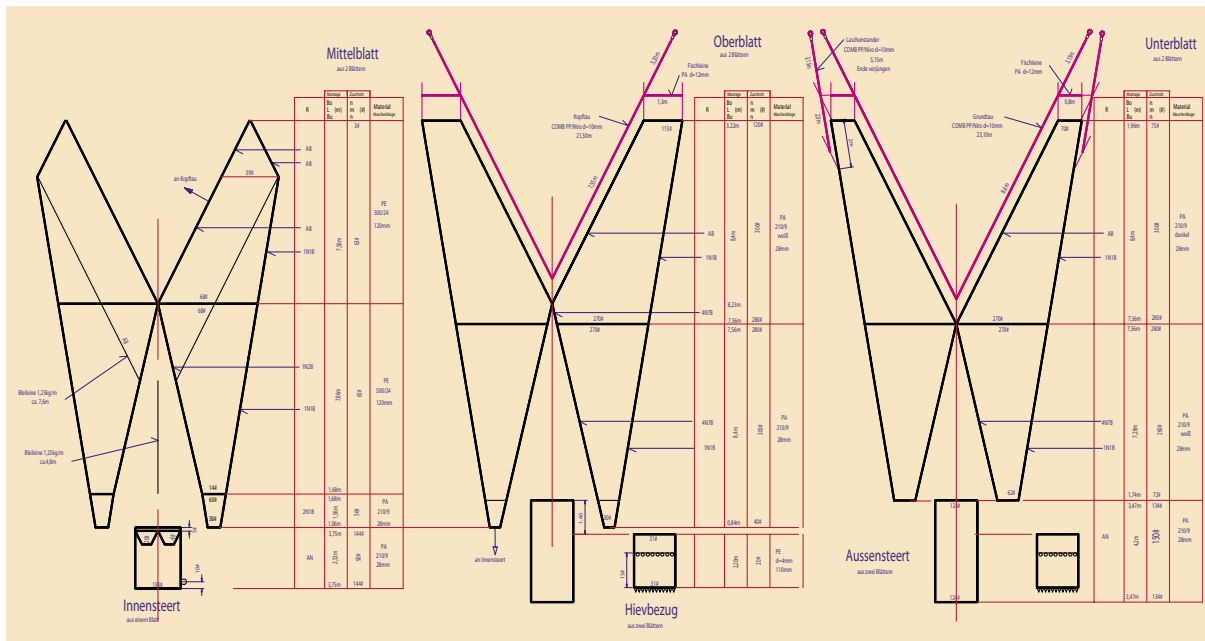
Abbildung 2: Maßstäbliche Fertigungszeichnung des Aalselektionstrawls Version 3. (Zeichnung: Rehme) Figure 2: To scale construction drawing of the eel selection trawl version 3. (Drawing: Rehme)
