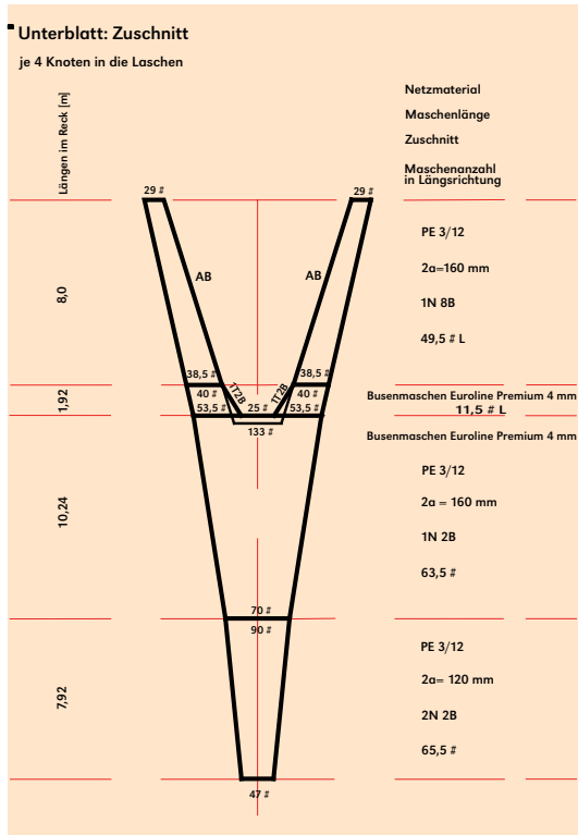
Abbildung 8: Zuschnitt des Unterblattes des reduzierten Grundsleppnetzes.
