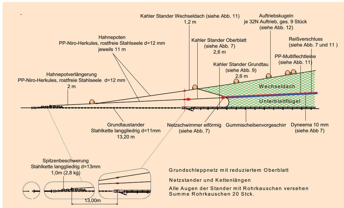
Abbildung 14: Netzstander des reduzierten Grundschieppnetzes mit Wechseldach.
