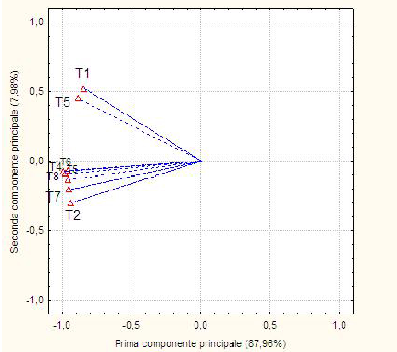
Fig. 45: Analisi delle componenti principali per il totale delle stazioni di monitoraggio nel 2009.
