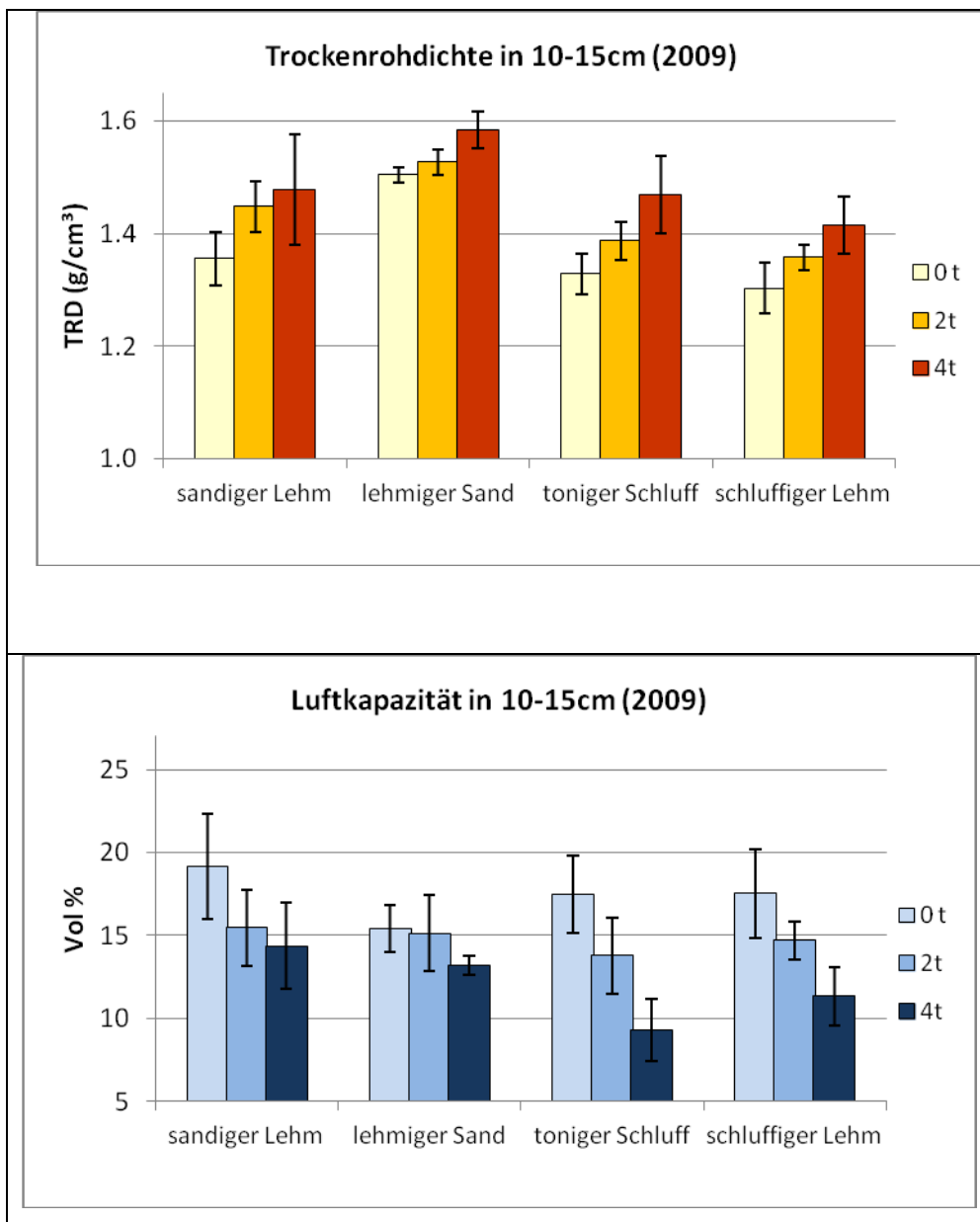
Abb1: Trockenrohdichte und Luftkapazität in einer Tiefe von 10-15 cm im Jahr 2009 auf allen vier Versuchsstandorten im unbelasteten Zustand (0 t) und nach Überrollung mit 2,6 t und 4,6 t (Mittelwerte aus vier Wiederholungen \pm Standardfehler).
