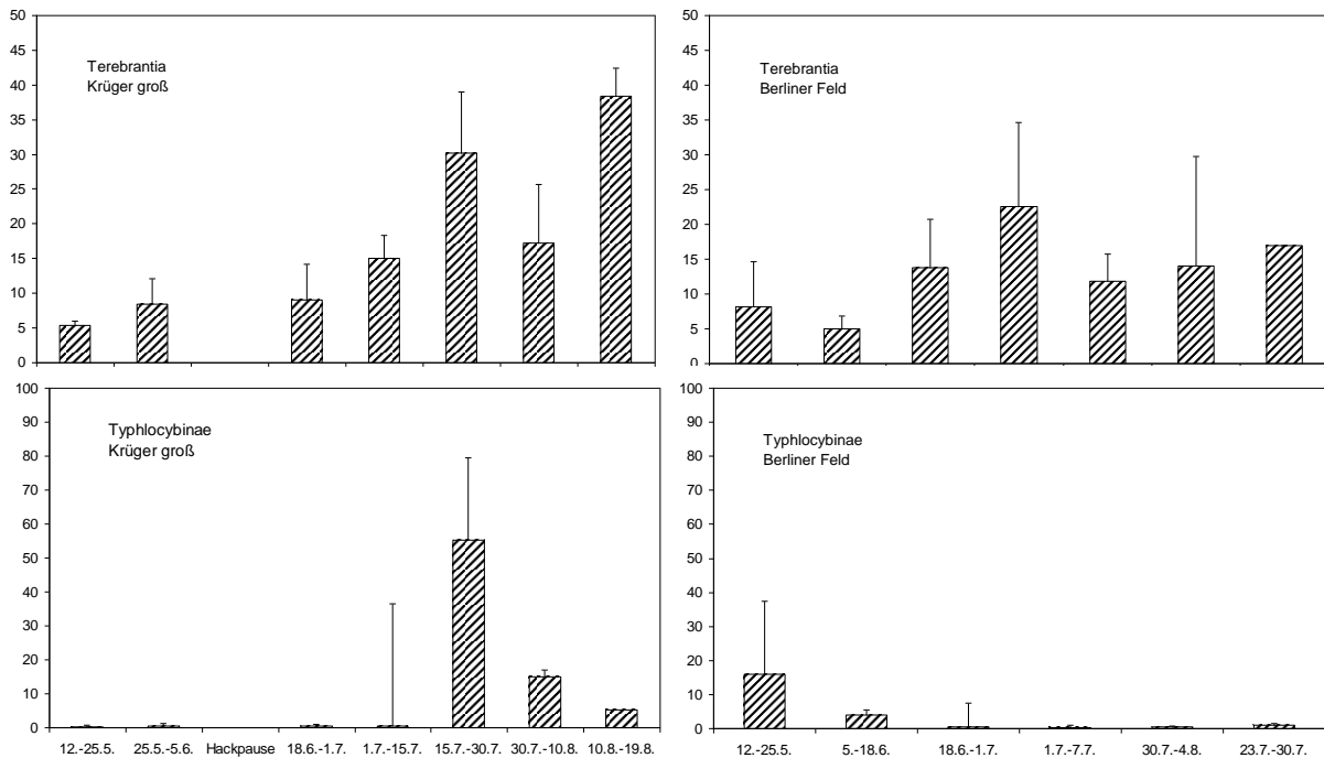
Abb. 5: Mittlere Fangsummen kleinwüchsiger Terebrantia und von Typhlocybinae (Blattzikaden) in den Bodenelektoren (n = 5) auf den Freitaler Salbeikulturen „Krüger groß“ und „Berliner Feld“. („Krüger groß“ 10.-19.8. n = 3, Berliner Feld 23.-30.7. n = 1). Beachte die verschiedene Skalierung der Y-Achse. 2009
