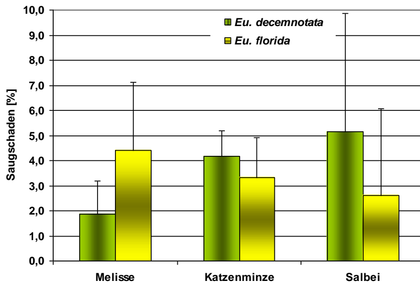
Abbildung 10 Saugschaden/Blatt [%] (Mittelwert \pm Standardabweichung, n = 5, 2 Versuche) von Eupertyx decemnotata und Eu. florida auf verschiedenen Wirtspflanzen drei Wochen nach dem Ansetzen von 90 adulten Zikaden und der Entwicklung unterschiedlicher Larvenzahlen (vgl. Abb. 9).
