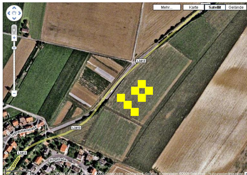
Abbildung 1 Schematische Darstellung der Gelbtafel Standorte auf einem 3-jährigen Melisseschlag in Habitzheim zum Zeitpunkt des zweiten Aufstelltermins (04.09.10). Versuch zur Erfassung der natürlichen Gegenspieler von Blattzikaden.
