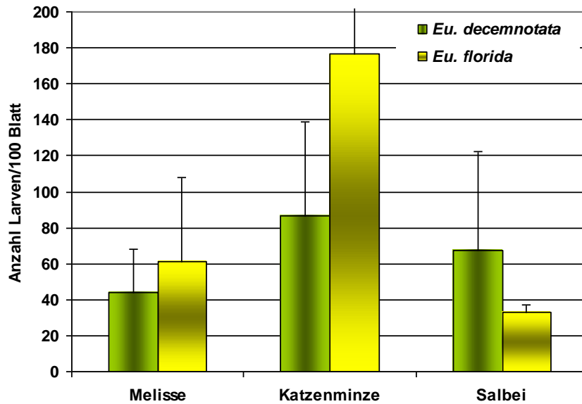
Abbildung 9 Anzahl Larven/100 Blatt (Mittelwert \pm Standardabweichung, n = 5, 2 Versuche) von Eupertyx decemnotata und Eu. florida auf verschiedenen Wirtspflanzen drei Wochen nach dem Ansetzen von 90 adulten Zikaden.
