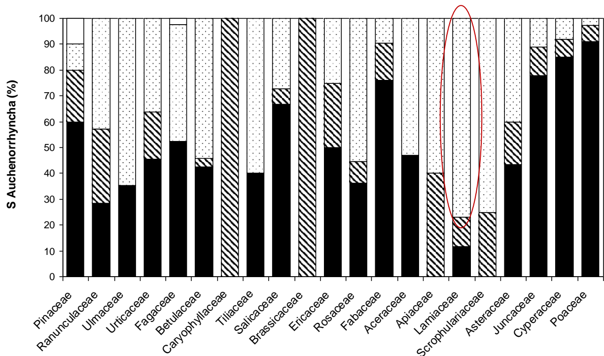
Abb. 11: Nahrungsressourcen von Zikaden der Gefäßpflanzenfamilien Deutschlands (ohne Überwinterer auf Pinaceae). Dargestellt sind nur Familien mit mehr als 5 Zikadenarten oder mehr als 100 Pflanzenarten. Schwarz = Phloem, schraffiert = Xylem, gepunktet = Mesophyll, weiß = Pilze. Nach Nickel (2003).
