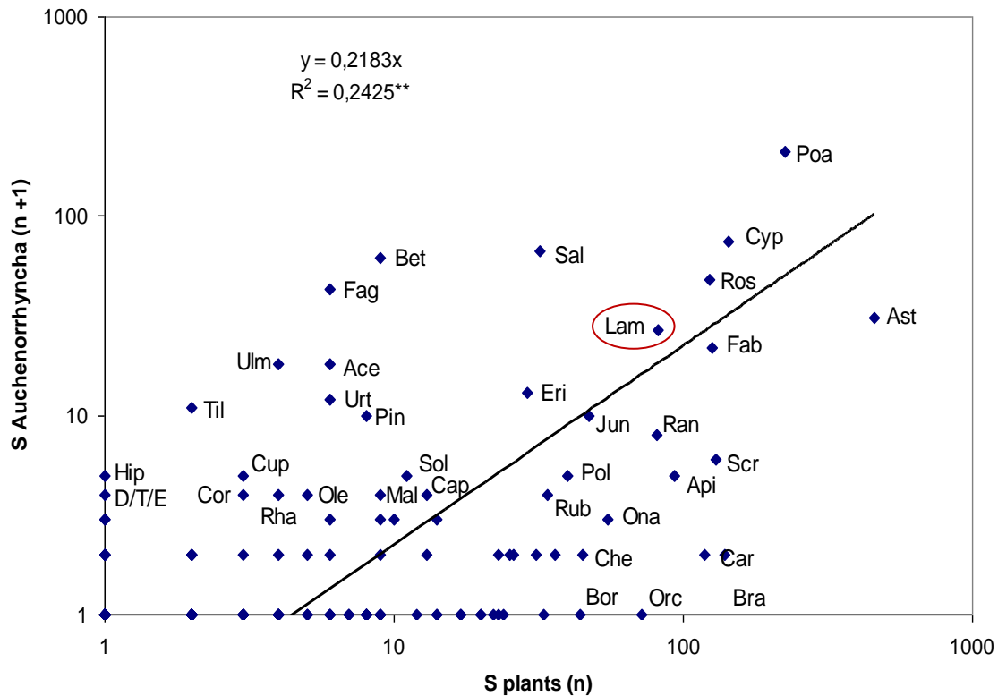
Abb. 10: Beziehung zwischen den Artenzahlen der Pflanzenfamilien und ihrer Zikaden in Deutschland. Dargestellt sind nur Familien mit mehr als 2 Zikadenarten oder mehr als 40 Pflanzenarten: Ace = Aceraceae, Api = Apiaceae, Ast = Asteraceae, Bet = Betulaceae, Bor = Boraginaceae, Bra = Brassicaceae, Cap = Caprifoliaceae, Car = Caryophyllaceae, Che = Chenopodiaceae, Cor = Cornaceae, Cup = Cupressaceae, Cyp = Cyperaceae, D/T/E = Dennstaedtiaceae/Taxaceae/Elaeagnaceae, Eri = Ericaceae, Fab = Fabaceae, Fag = Fagaceae, Hip = Hippocastanaceae, Jun = Juncaceae, Lam = Lamiaceae, Mal = Malvaceae, Ole = Oleaceae, Ona = Onagraceae, Orc = Orchidaceae, Pol = Polygonaceae, Pin = Pinaceae, Poa = Poaceae, Ran = Ranunculaceae, Rha = Rhamnaceae, Ros = Rosaceae, Rub = Rubiaceae, Sal = Salicaceae, Scr = Scrophulariaceae, Sol = Solanaceae, Til = Tiliaceae, Ulm = Ulmaceae, Urt = Urticaceae. Nach Nickel (2003).
