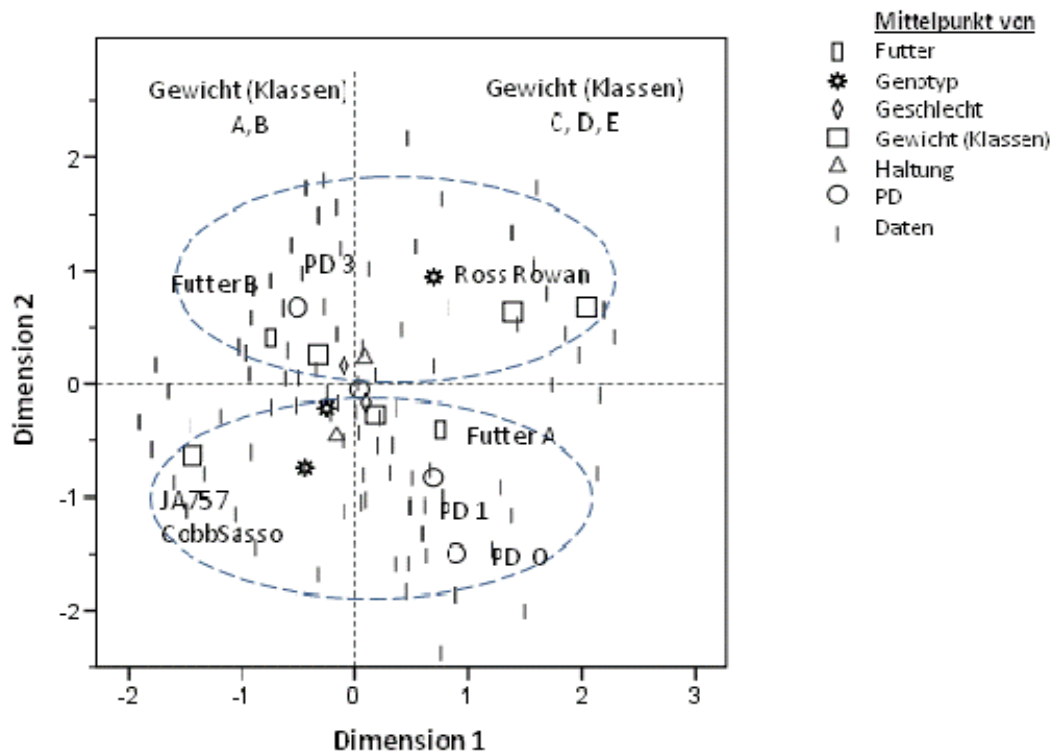
Abbildung 3: Streudiagramm der Dimensionen 1 und 2 der Hauptkomponentenanalyse im Durchgang 2 für die Variablen Genotyp, Futter, Haltung, Geschlecht, Lebendgewichtsklasse (Klassenbreite 300 g) und Pododermatitis bei Masthähnchen nach einer Mastdauer von 56 Tagen
