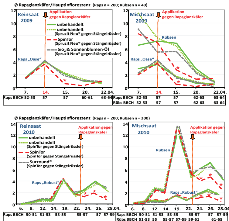
Abb. 2: Zeitlicher Verlauf des Befalls mit Meligethes aeneus in Abhängigkeit der Anbau- und Pflanzenschutzmittelvarianten; * = signifikant für \alpha = 5\% Wilcoxon Test
