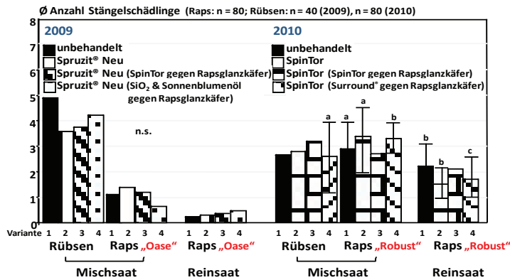
Abb. 1: Einfluss der Anbau- und Pflanzenschutzmittelvariante auf den Befall mit Cetorhynchus spp. ; n.s. = nicht signifikant für \alpha = 5\% Wilcoxon Test
