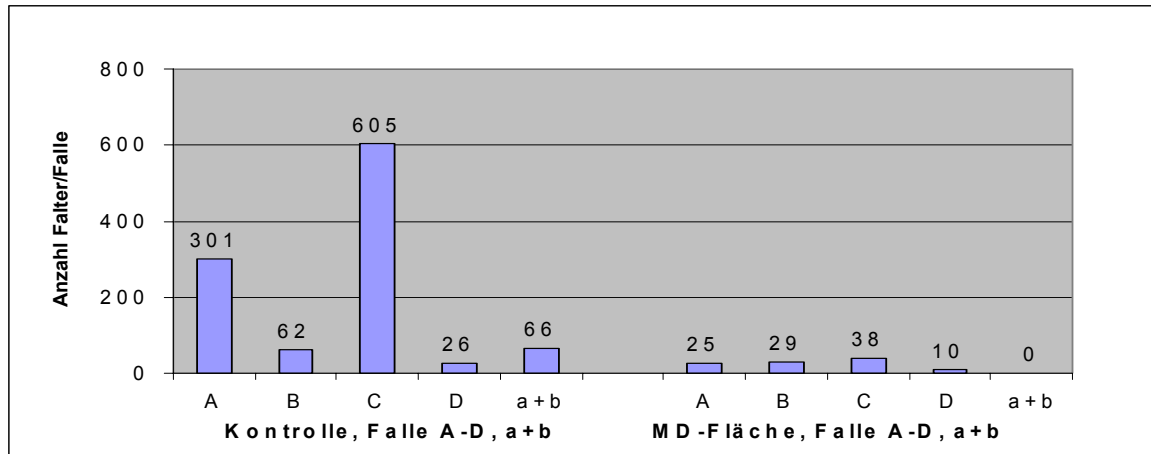
Abb. 1: Fangsummen in den Fallenpositionen A-D außerhalb des Feldes und im Bestand aufgestellten Fallen a, b, jew. als Summe Tripheron ® + Pherobank ® -Falle. Feldversuch Guntershausen (2000).
