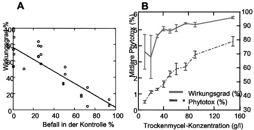
Fig. 1A: Einfluss von PEN auf den Krankheitsbefall von Tomate durch Phytophthora infestans . Der Wirkungsgrad nimmt bei zunehmendem Befallsdruck ab. Jeder Punkt repräsentiert den Mittelwert von 6 Wiederholungen. Fig 1B: Einfluss der Konzentration von PEN auf den Befall von Tomaten durch Phytophthora infestans und auf die Ausprägung von Phytotoxizität.
