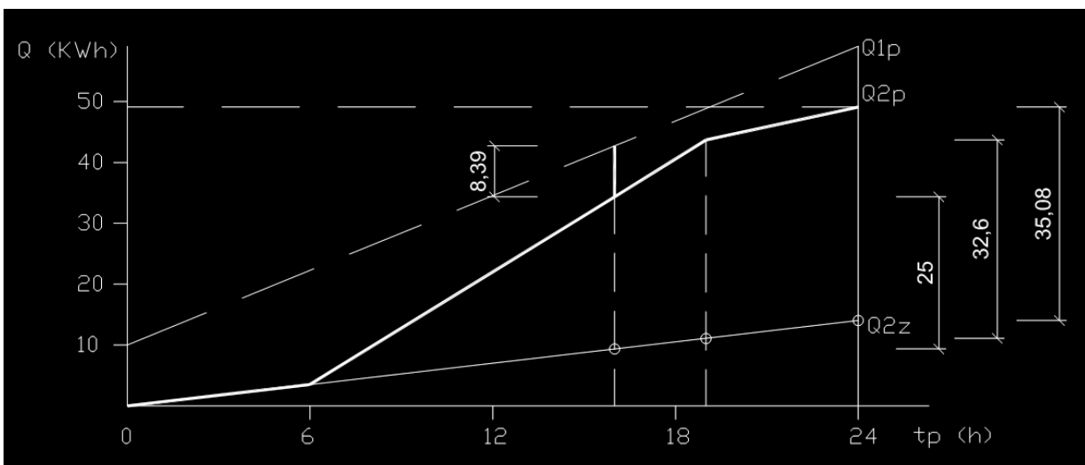
Obr.1 Křivka odběru
