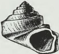
Trochonema 1X
