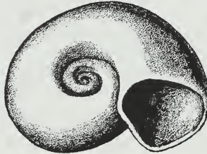
Maclurites 1X
