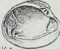
Venus 1/3X
