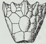
Eucalyptocrinus 2/3X
