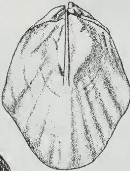
Pentamerus 1/2 X
