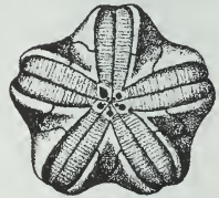
Pentremites 2/3X
