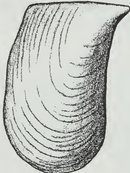
Myalina 2/3X
