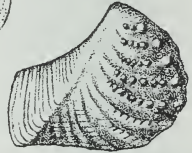
Trigonina 2/3X
