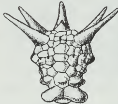
Doryocrinus 1X
