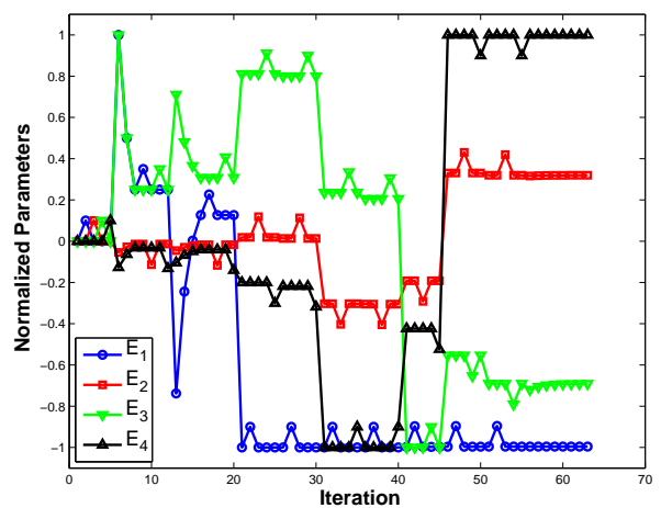
(d) Parameters Convergence
