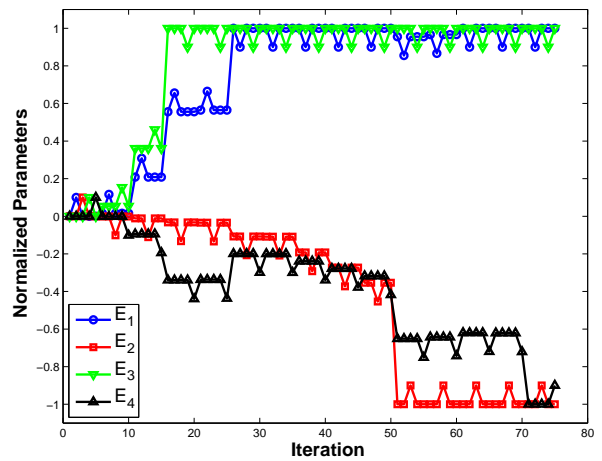
(b) Parameters Convergence
