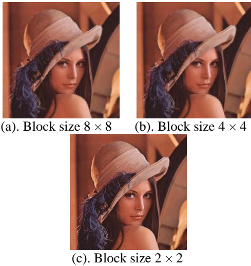
Fig.6. Lena
