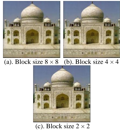
Fig.9. Taj Mahal
