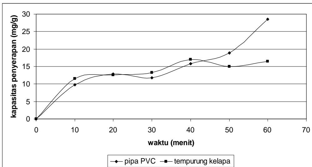
Gambar 11. Kapasitas penyerapan logam kromium oleh biofilm P. putida dengan medium pendukung tempurung kelapa dan pipa PVC.
